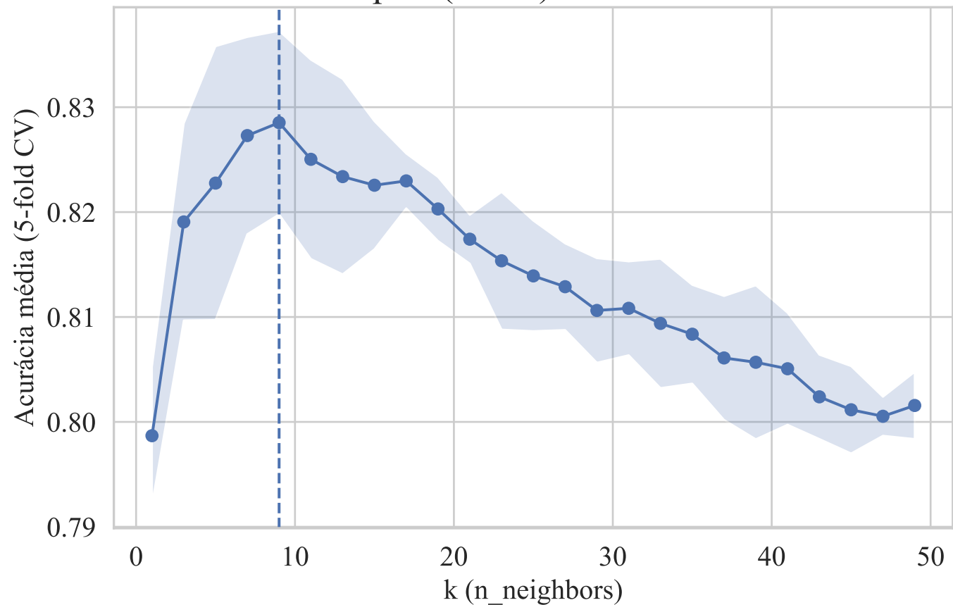
Elbow plot (k-NN) — melhor k = 9
