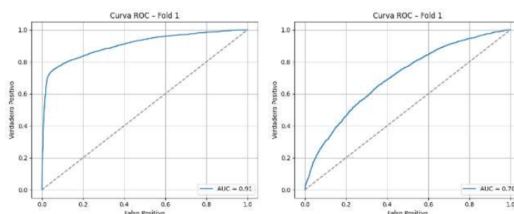
Figura 1. Curvas ROC validação externa LightGBM para casos confirmados (esquerda) e para severidade (direita).
