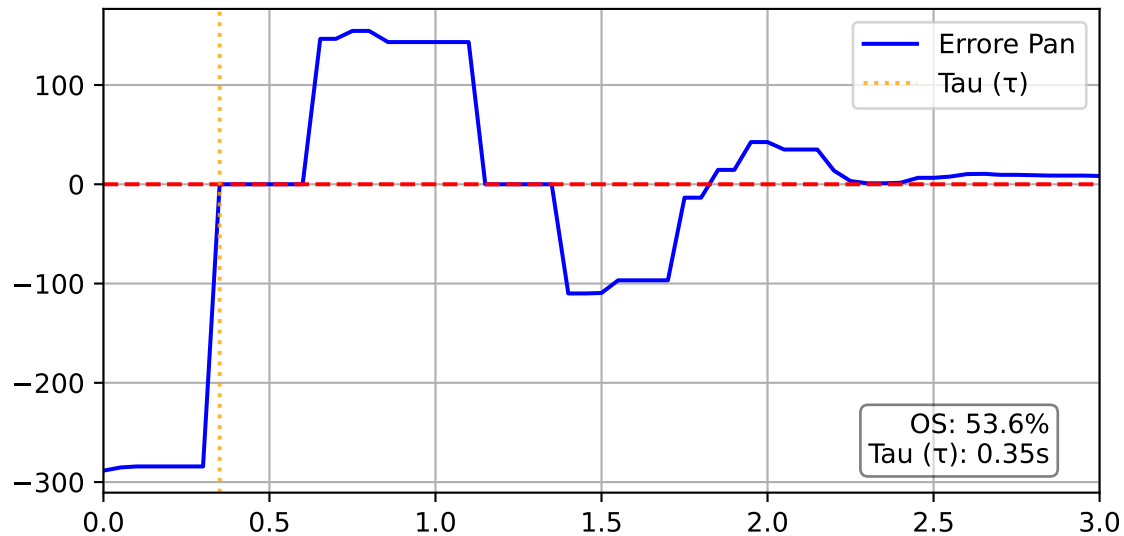
Risposta Pan
