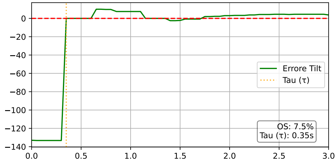
Risposta Tilt
