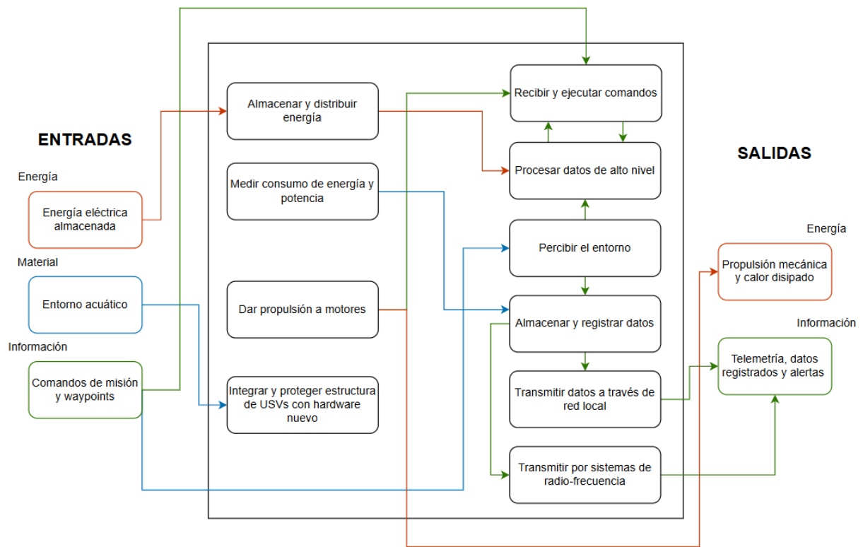
Figura 3.4: Descomposición funcional de primer nivel del sistema a diseñar
