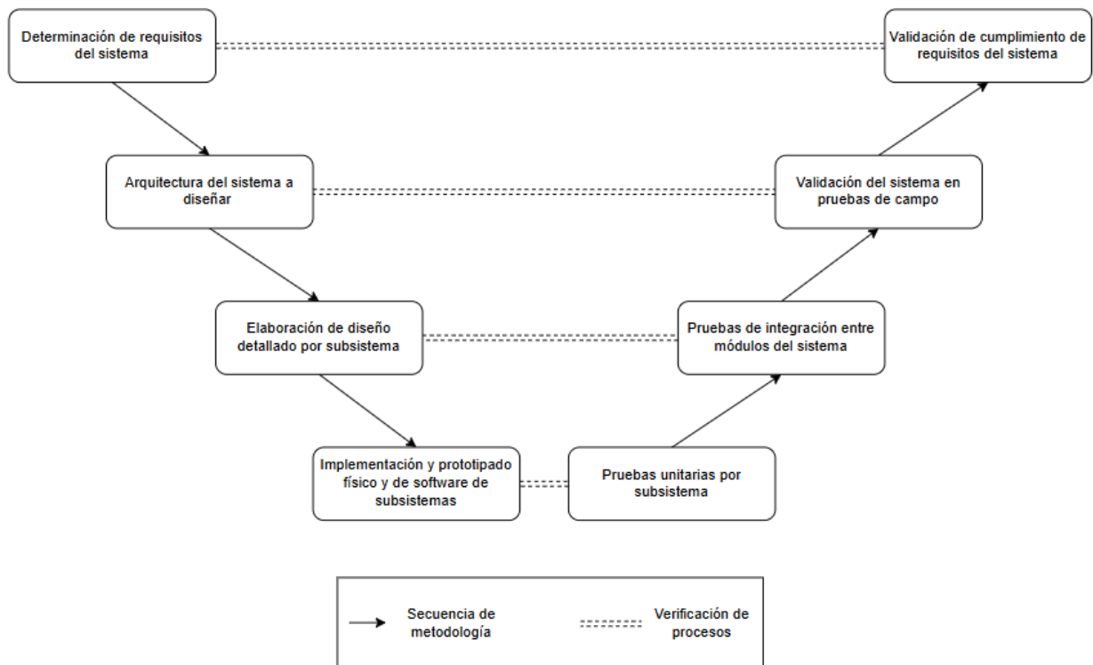
Figura 3.1: Diagrama de flujo de la metodología en V [8] [9]
