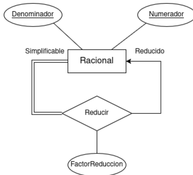
Figura 3: Diagrama E/R que representa los números racionales.
