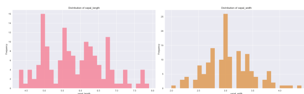
Figura 1. Distribuição das características sepal_length e sepal_width .
