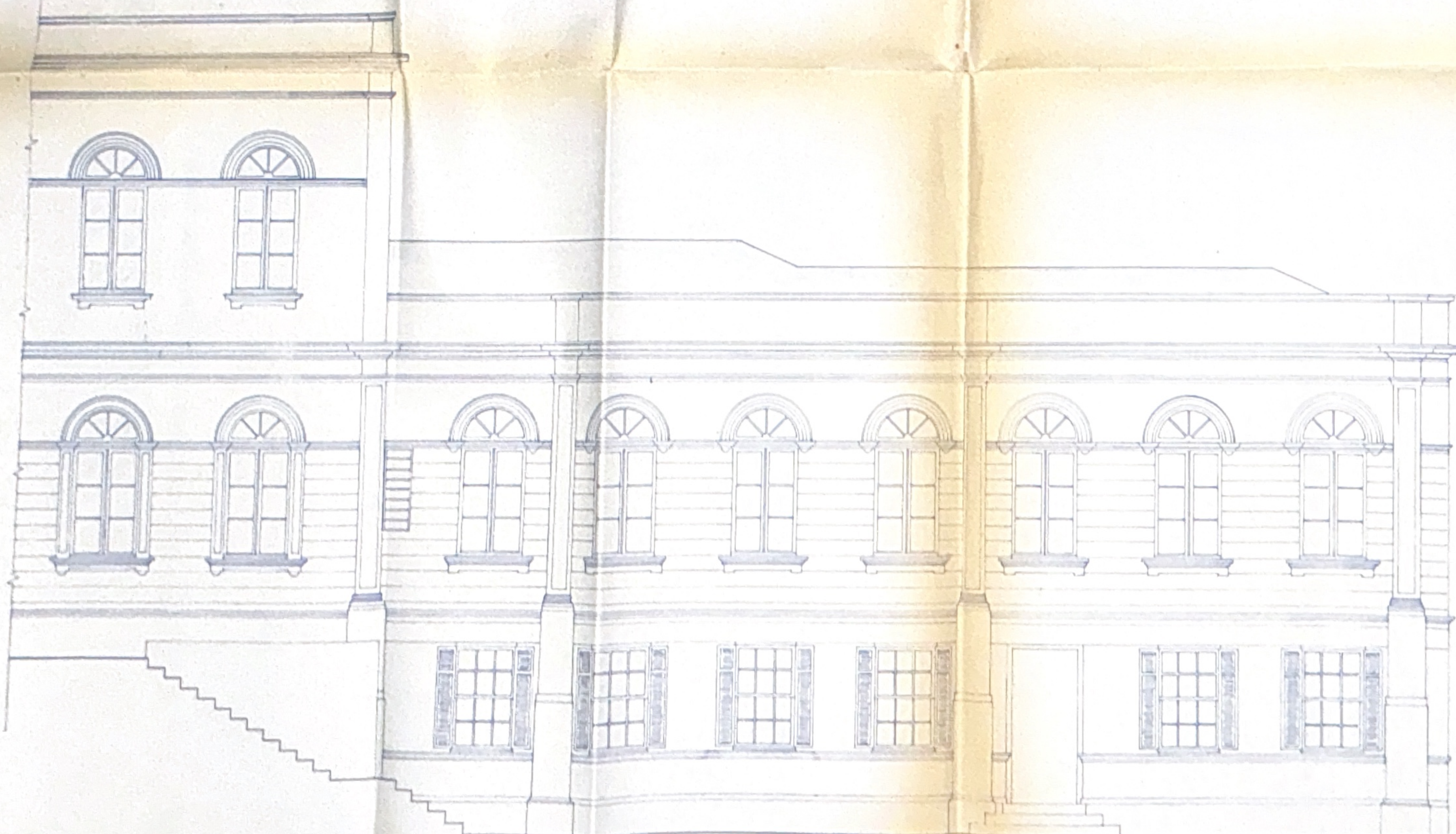
FACHADA PARCIAL DA RUA 13 DE MAIO — ESCALA 1:50
