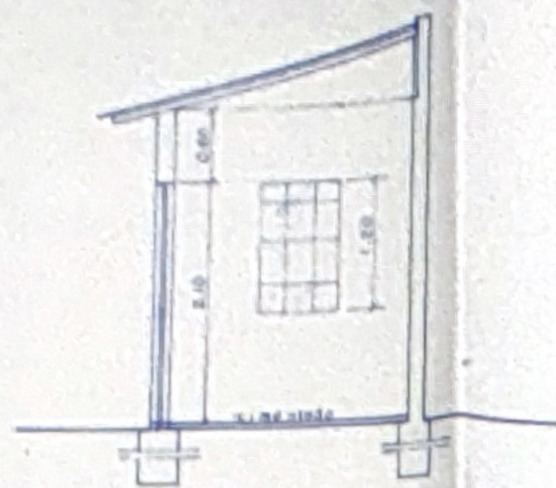
CORTE C-D — ESCALA 1:50
