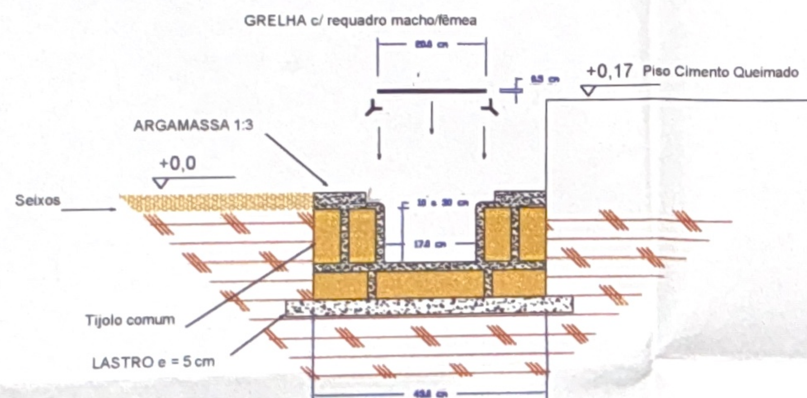
Detalhe da canaleta de drenagem esc. 1:10
