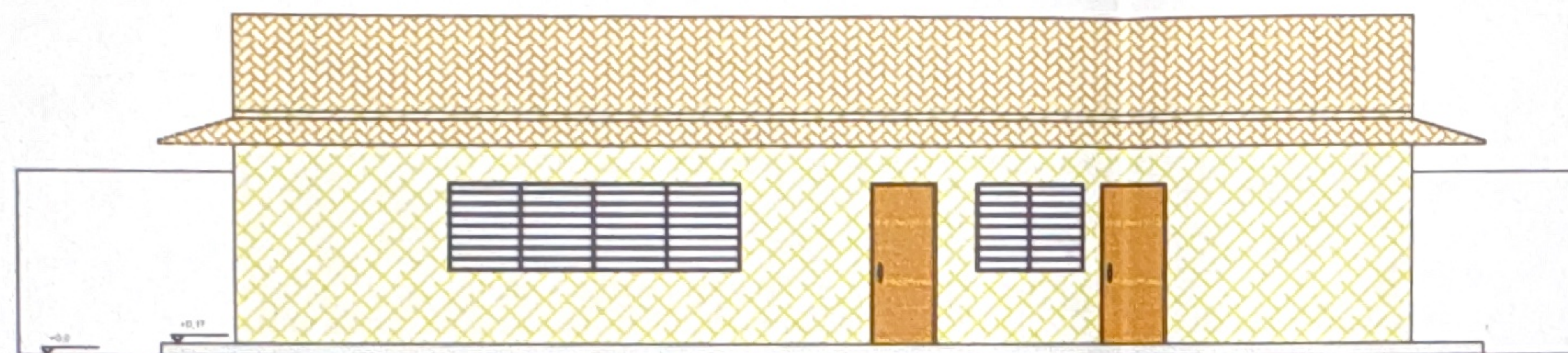
Fachada Frontal esc. 1:100
