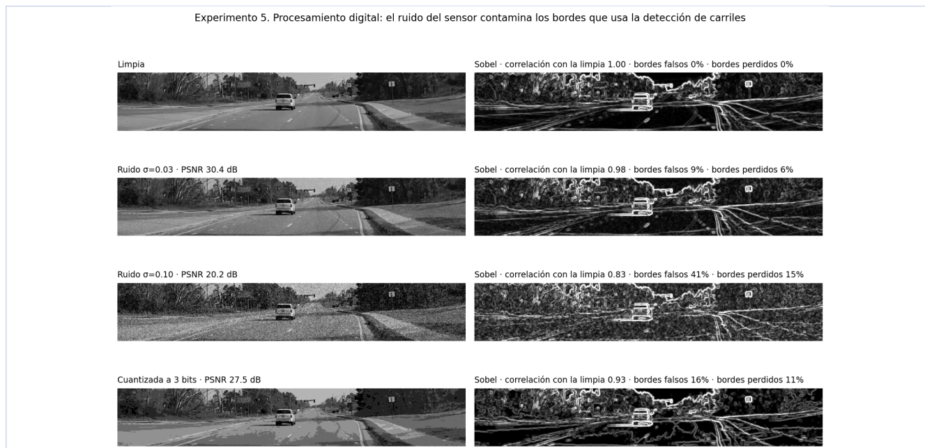
Figura 6. Tramo de carretera en gris (izquierda) y su mapa de bordes de Sobel (derecha) con distintas degradaciones del sensor.
