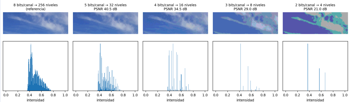
Figura 3. Cielo con degradado suave cuantizado a distinto número de bits por canal, con su histograma.
