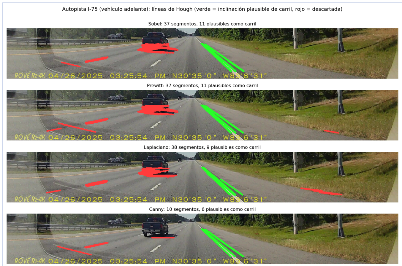
Figura 2. I-75: segmentos de Hough sobre el mapa de bordes de cada operador. Verde: inclinación plausible de carril (entre 20° y 80° respecto a la horizontal); rojo: descartado. El vehículo de adelante genera segmentos horizontales descartados.
