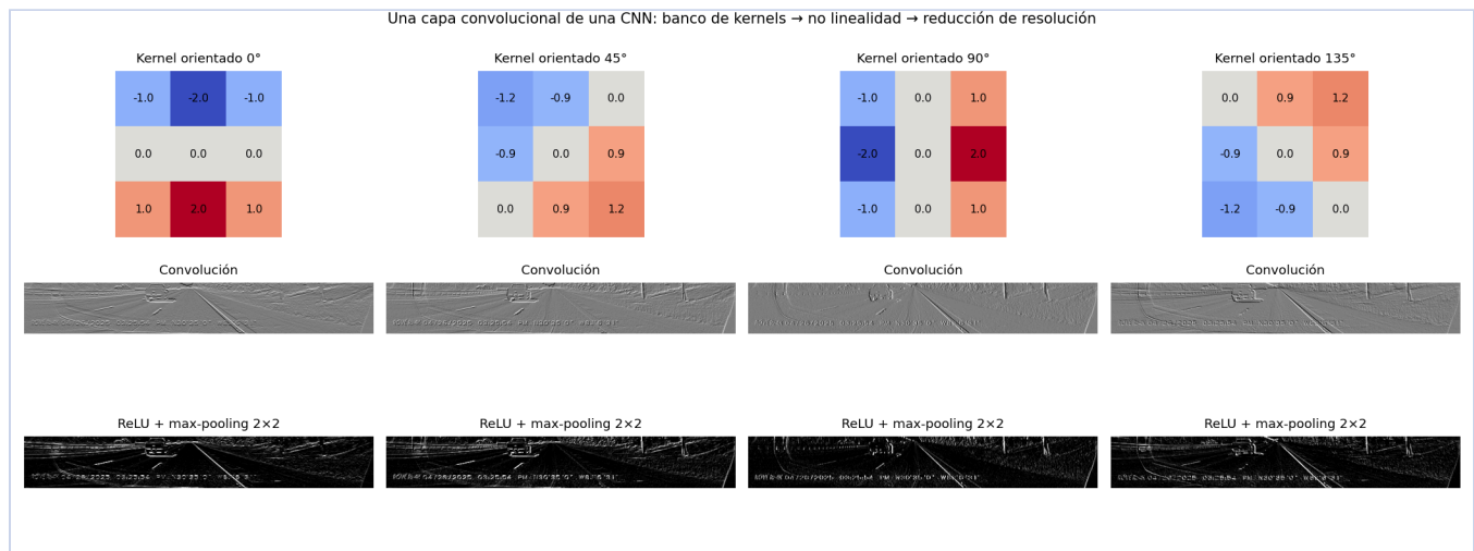
Figura 5. Una capa convolucional con un banco de cuatro kernels orientados (derivados del Sobel), ReLU y max-pooling 2x2 sobre la franja de la calzada de la I-75. Los kernels se giraron con interpolación, por eso algunos coeficientes no son enteros.
