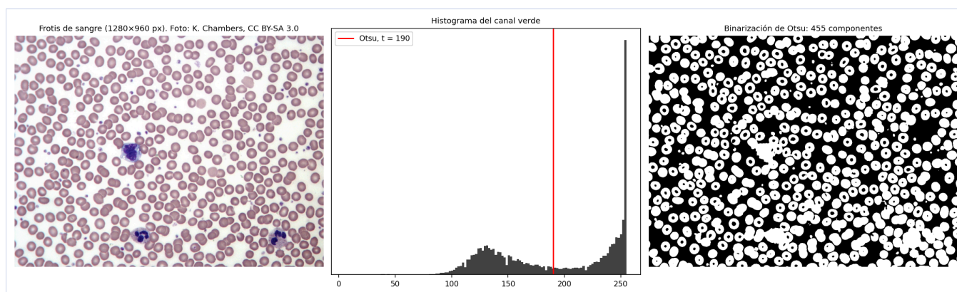
Figura 1. Frotis original, histograma del canal verde con el umbral de Otsu y binarización resultante.
