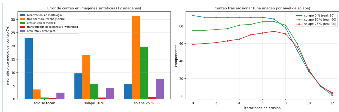
Figura 6. Izquierda: error medio del conteo por método y nivel de traslape. Derecha: conteo tras erosionar (una imagen por nivel de traslape).
