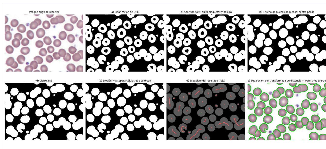
Figura 2. Etapas del procesamiento sobre un recorte: (a) binarización, (b) apertura, (c) relleno de huecos, (d) cierre, (e) erosión, (f) esqueleto y (g) separación por transformada de distancia y watershed.
