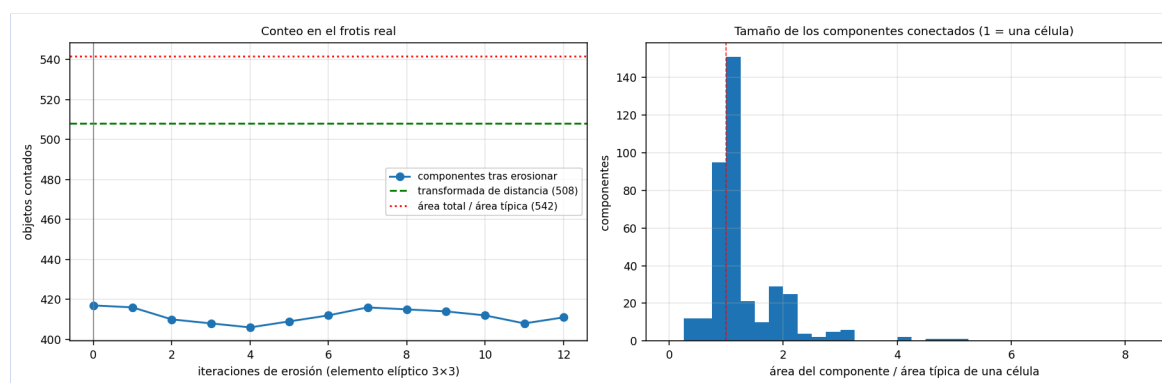
Figura 3. Izquierda: conteo en el frotis real según las iteraciones de erosión, comparado con la transformada de distancia y con el área total dividida entre el área típica. Derecha: tamaño de cada componente conectado respecto del área típica.
