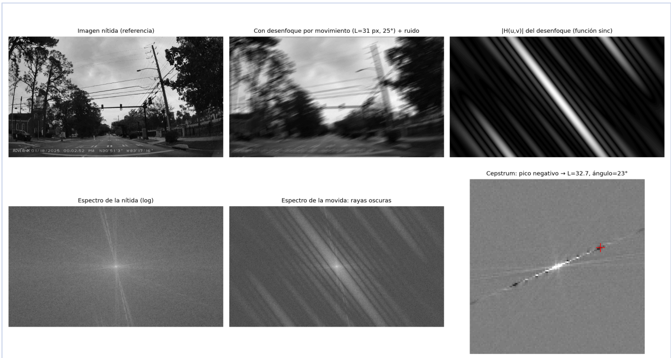
Figura 1. Imagen nítida y movida (foto: M. Rivera, CC0), transferencia H del desenfoque, espectros y cepstrum. Las rayas oscuras del espectro de la movida son los ceros del sinc, perpendiculares a la dirección del movimiento.
