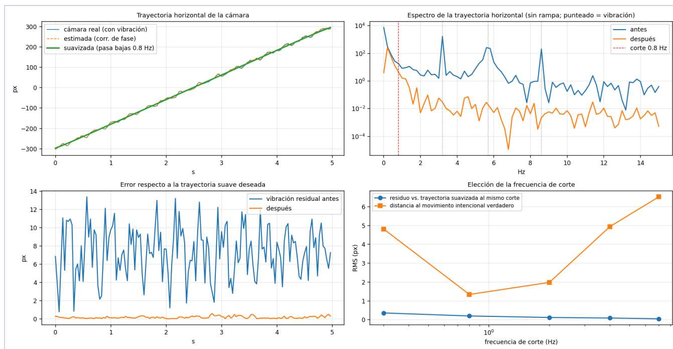
Figura 3. Arriba a la izquierda: trayectoria horizontal real, estimada y suavizada. Arriba a la derecha: espectro de la trayectoria sin la rampa, antes y después; los tres picos de la vibración desaparecen. Abajo: error respecto de la trayectoria suave deseada y elección de la frecuencia de corte.
