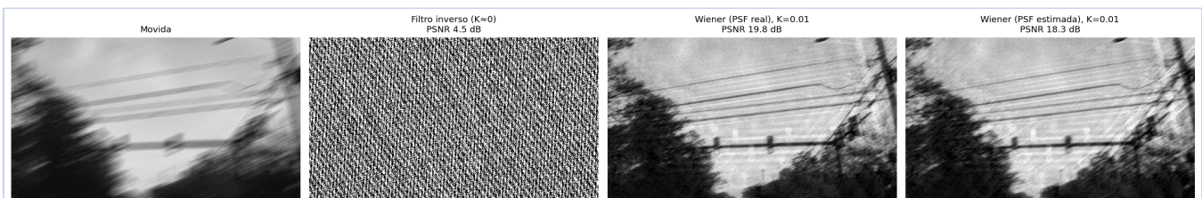
Figura 2. Recorte de la imagen movida y de las restauraciones: filtro inverso, Wiener con la función de desenfoque real y Wiener con la estimada por cepstrum.
