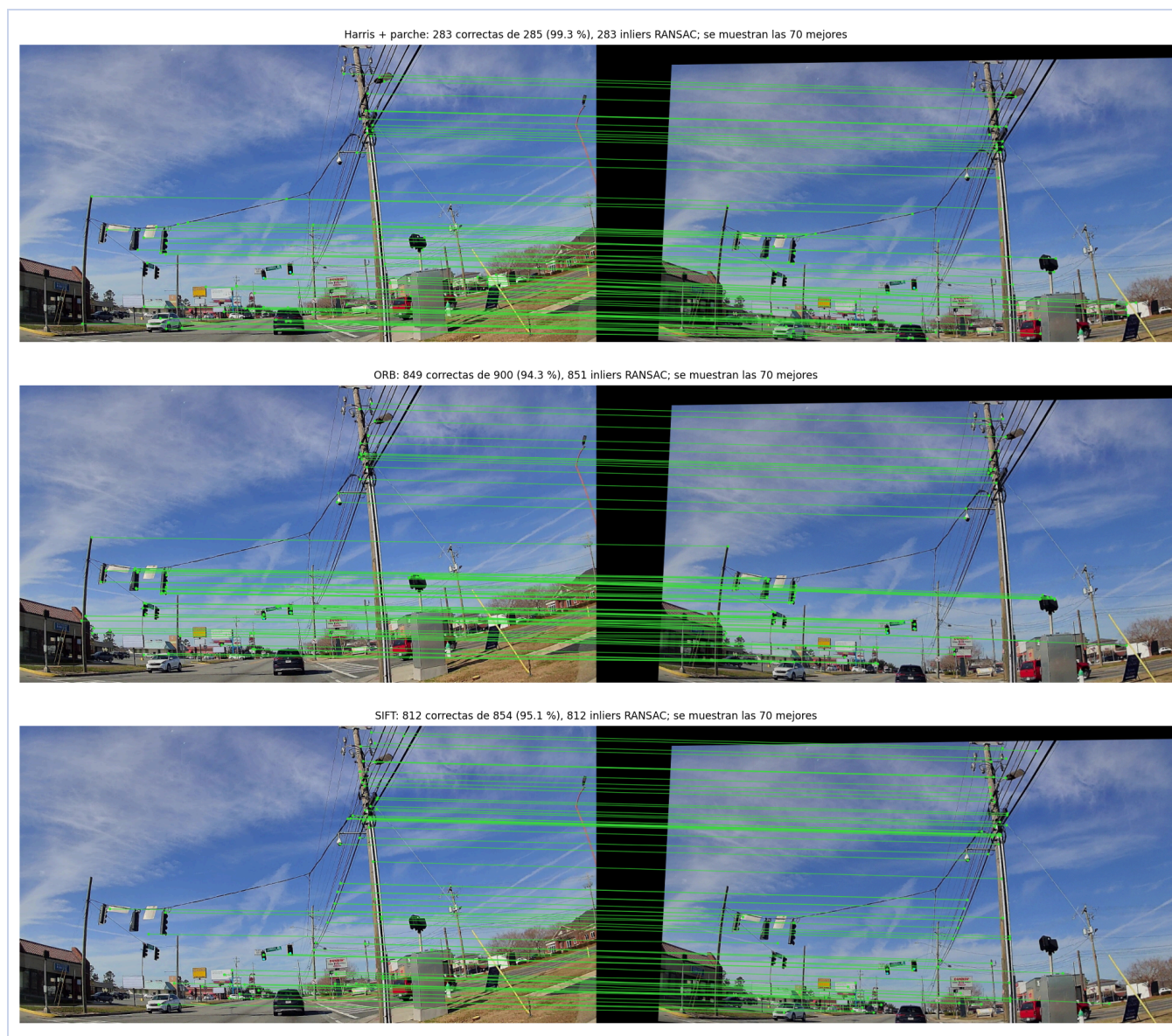
Figura 3. Correspondencias entre la vista 1 (izquierda) y la vista 2 (derecha) con Harris + parche, ORB y SIFT. Verde: correcta según la verdad; rojo: errónea (no aparece ninguna entre las 70 mejores).
