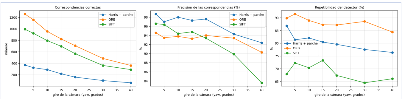
Figura 4. Efecto del giro de la cámara (yaw) sobre el número de correspondencias correctas, su precisión y la repetibilidad del detector.
