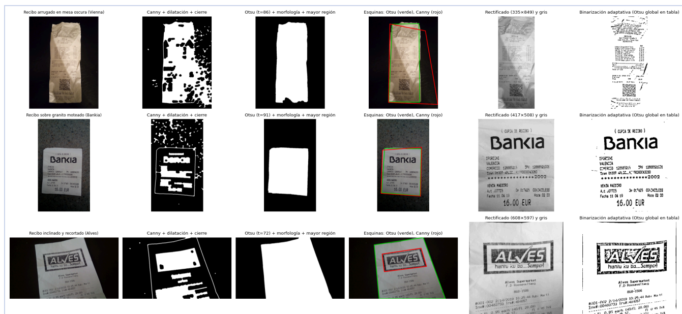
Figura 1. Etapas en cada recibo real (de izquierda a derecha): original, bordes de Canny con morfología, máscara de Otsu con morfología, esquinas detectadas por Otsu (verde) y Canny (rojo), documento rectificado en gris y binarización adaptativa.
