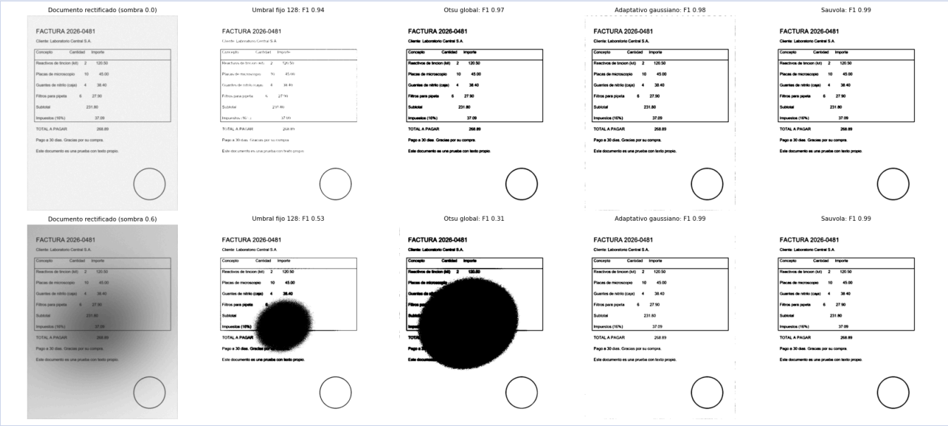
Figura 3. Binarización del documento rectificado (fila superior: sin sombra; inferior: sombra de 0.6) con umbral fijo, Otsu global, umbral adaptativo gaussiano y Sauvola.
