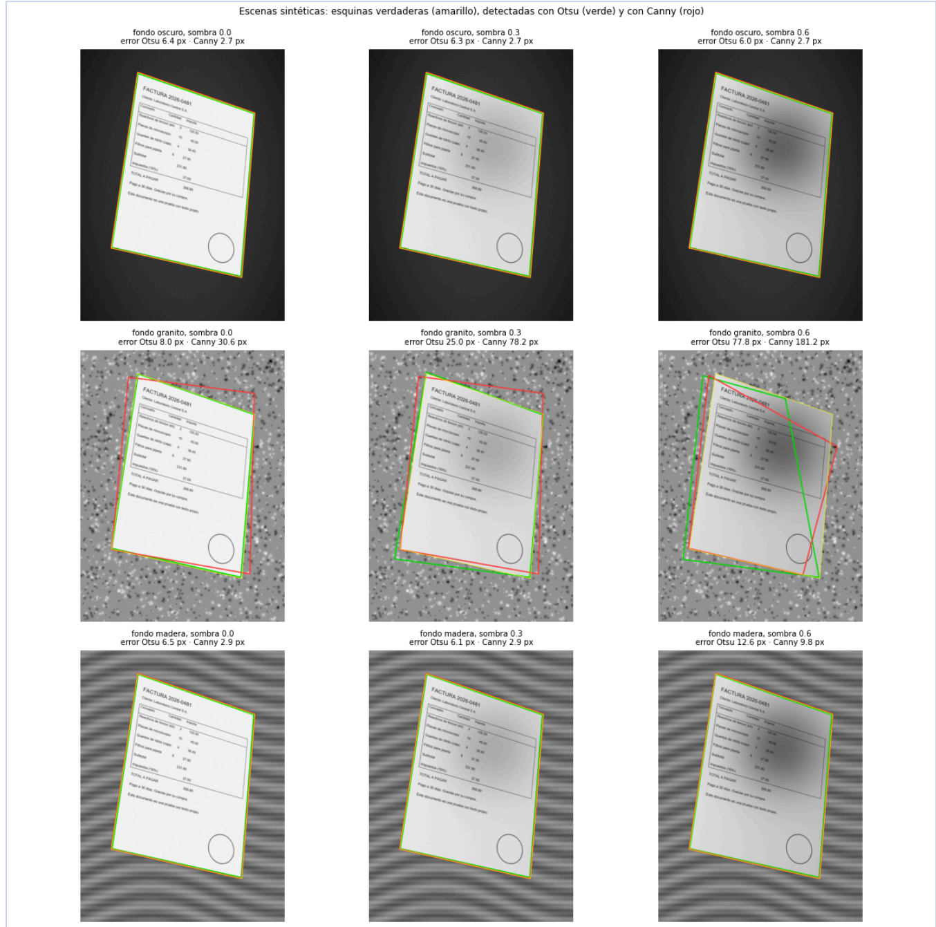
Figura 2. Escenas sintéticas: esquinas verdaderas (amarillo), detectadas con Otsu (verde) y con Canny (rojo), para cada fondo y nivel de sombra.
