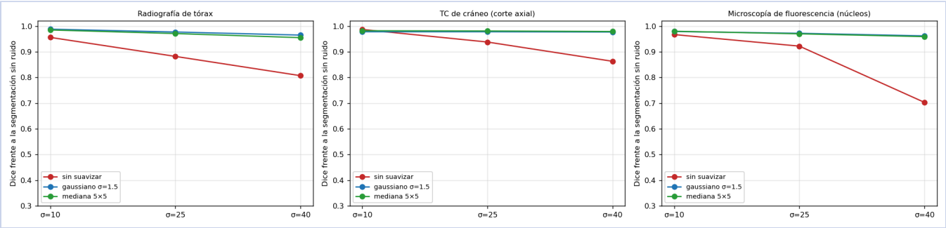
Figura 2. Coincidencia (Dice) entre la segmentación de una imagen con ruido y la de la imagen sin ruido, con y sin suavizado previo.
