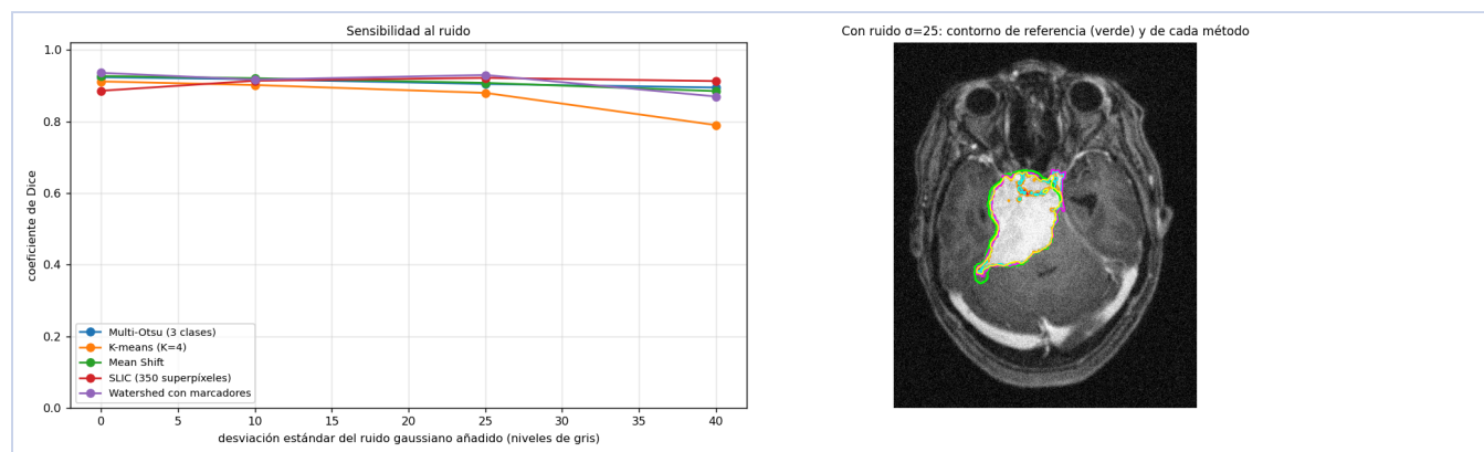
Figura 3. Izquierda: Dice en función del ruido añadido. Derecha: contornos de cada método con ruido \sigma = 25 .
