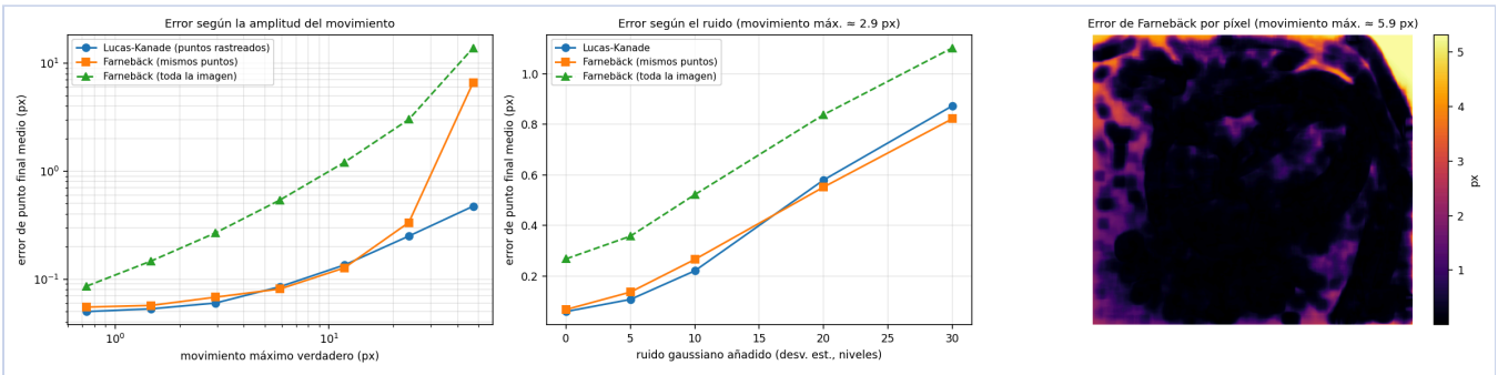
Figura 5. Error de punto final frente a un flujo verdadero conocido. Izquierda: según la amplitud del movimiento. Centro: según el ruido añadido. Derecha: error de Farneback por píxel.
