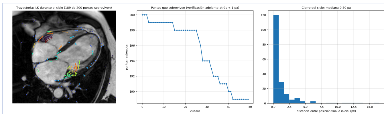
Figura 2. Izquierda: trayectorias de Lucas-Kanade durante el ciclo (color = desplazamiento máximo). Centro: puntos que sobreviven a la verificación adelante-atrás. Derecha: distancia entre posición final e inicial, que debería ser cero si el ciclo se cierra.
