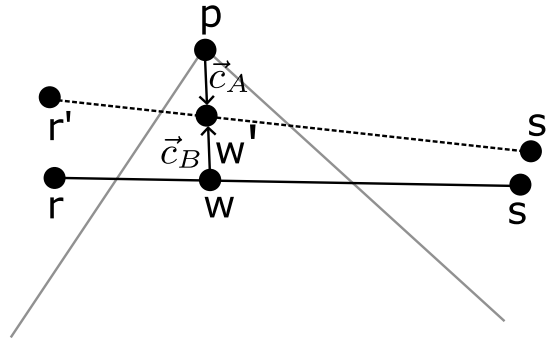
Figura 15 – Caso colisão vértice-aresta. Correção das posição para configuração válida. O vértice mais próximo de w sofre maior deslocamento, preservando a coerência geométrica da aresta. Fonte: Adaptado de (JAKOBSEN, 2001).
