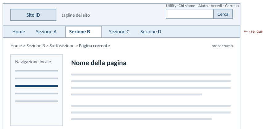
Schema originale: anatomia di una pagina con navigazione persistente, breadcrumb, nome della pagina e indicatore “sei qui”.
