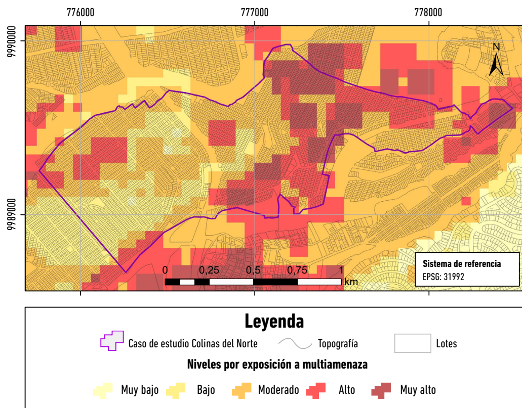
Figura 3. Nivel de multiamenaza en el barrio Colinas del Norte. Datos: MDMQ (2021); Secretaría de Planificación (2021).
