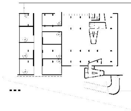
Figura 10: Edif. Walfrido Antunes (1956). Térreo e sobreloja com lojas - Proj. Waldecy Pinto.
