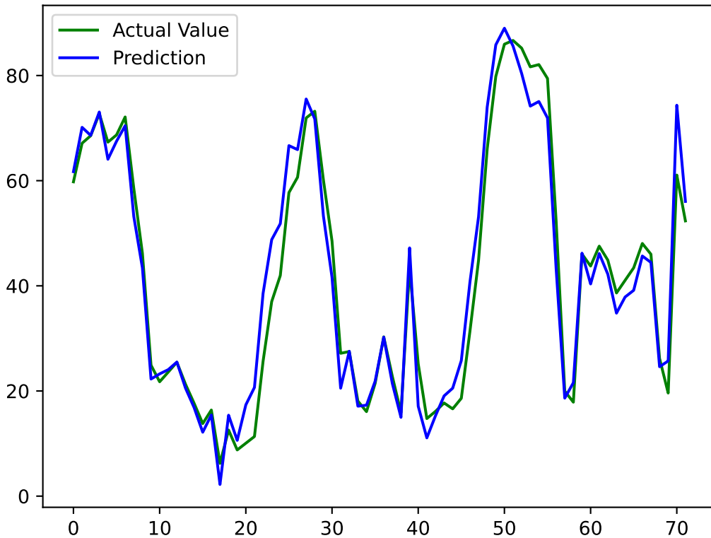
Predicted vs Actual Values
