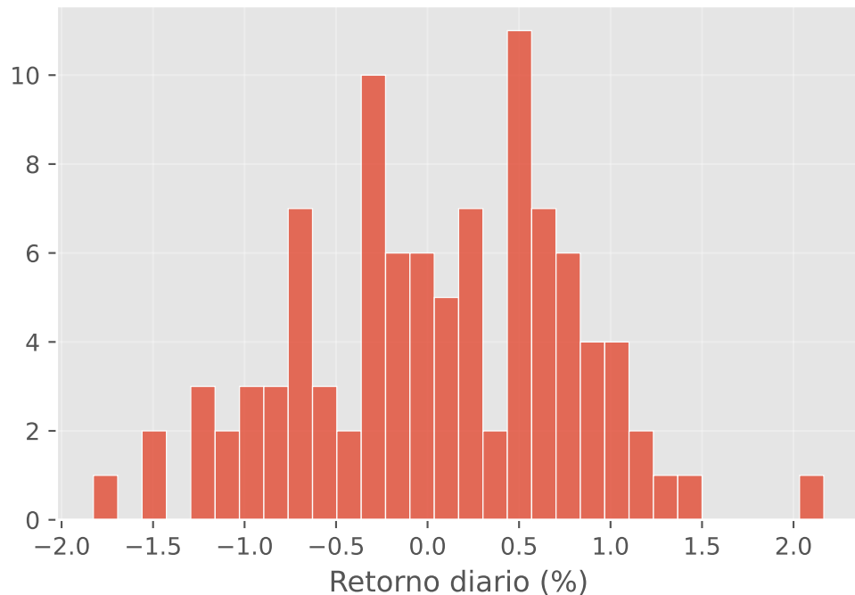
Histograma: la distribución de retornos
