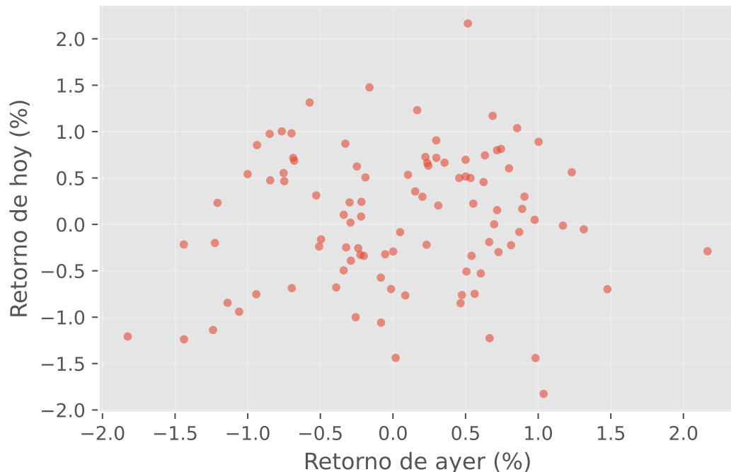
Dispersión: retorno vs. retorno anterior
