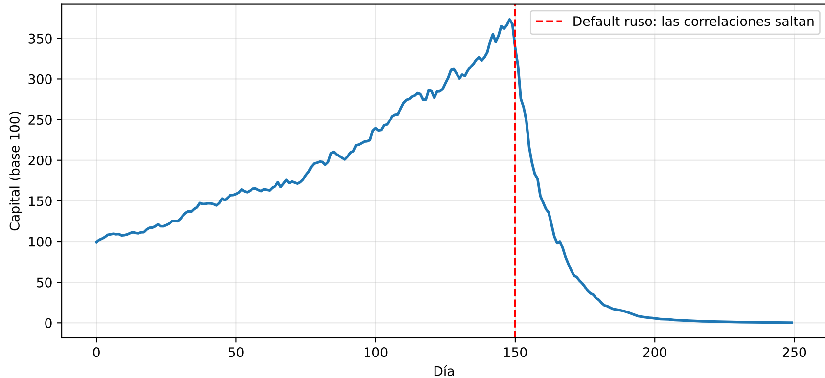
LTCM estilizado: 10 apuestas 'independientes' con apalancamiento 25:1
