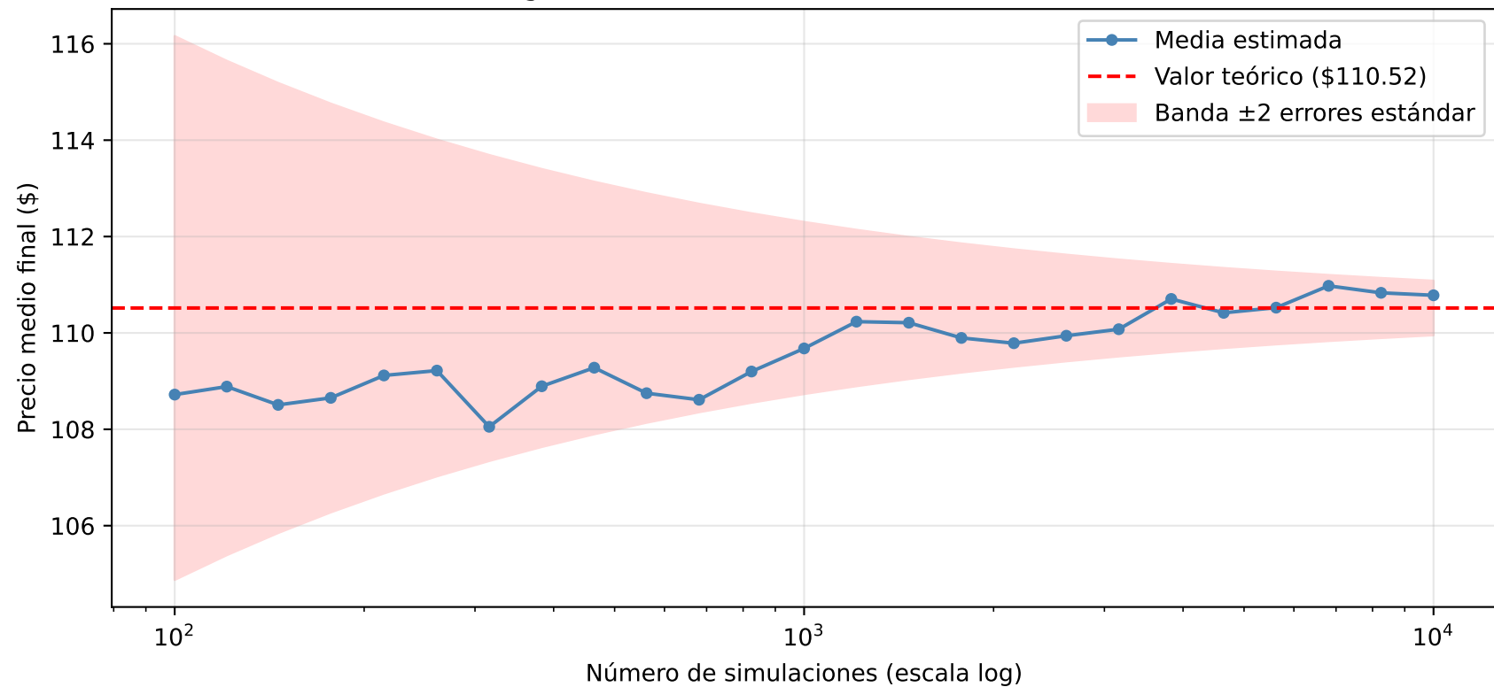
Convergencia de Monte Carlo: el error cae como 1/\sqrt{N}
