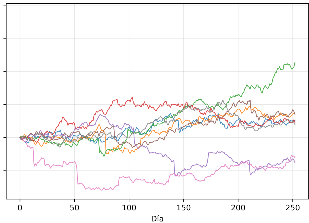
Merton (difusión + saltos)
