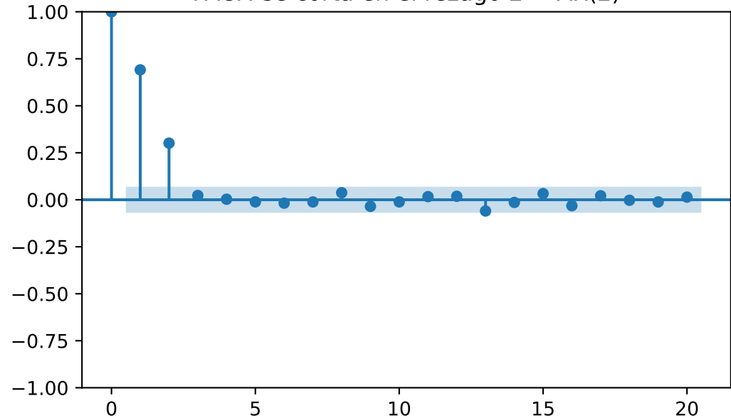
PACF: se corta en el rezago 2 \rightarrow AR(2)
