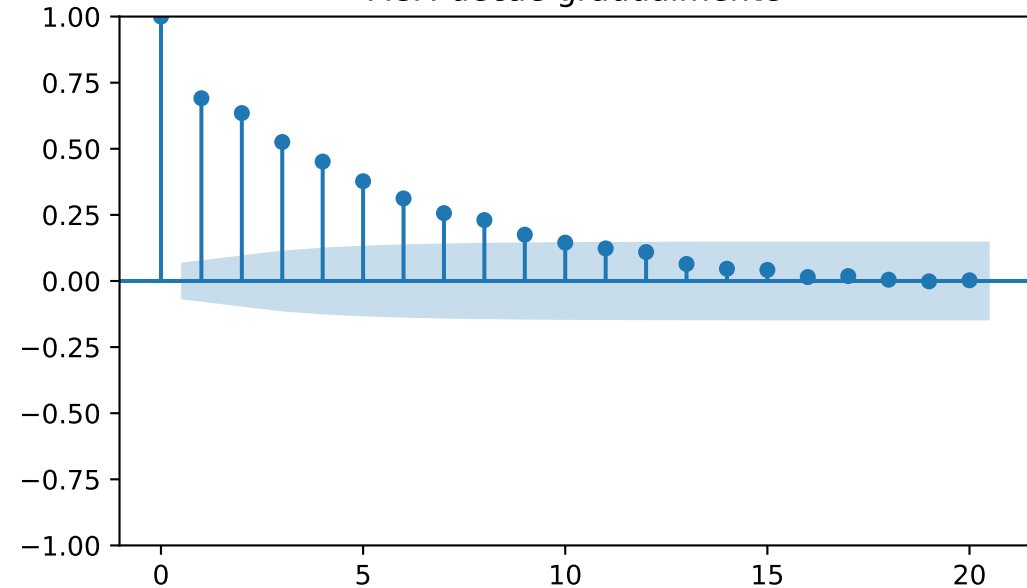
ACF: decae gradualmente
