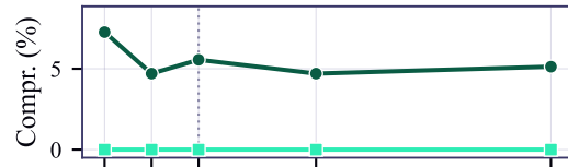
Catalog compression
