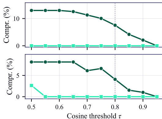
Catalog compression
