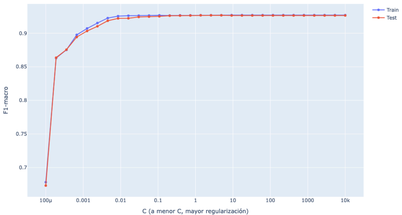
Figura 4. F1-macro en entrenamiento y prueba para distintos valores de C . Un valor menor de C implica una regularización más intensa.
