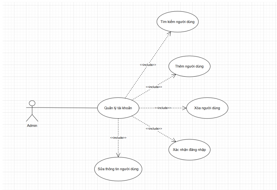
Hình 5: Biểu đồ phân rã ca sử dụng Quản lý tài khoản
