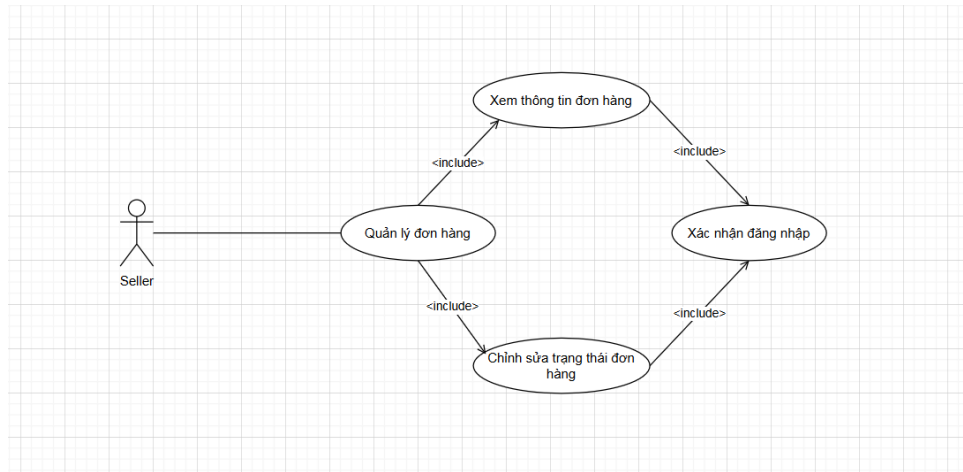
Hình 4: Biểu đồ phân rã ca sử dụng Quản lý đơn hàng
