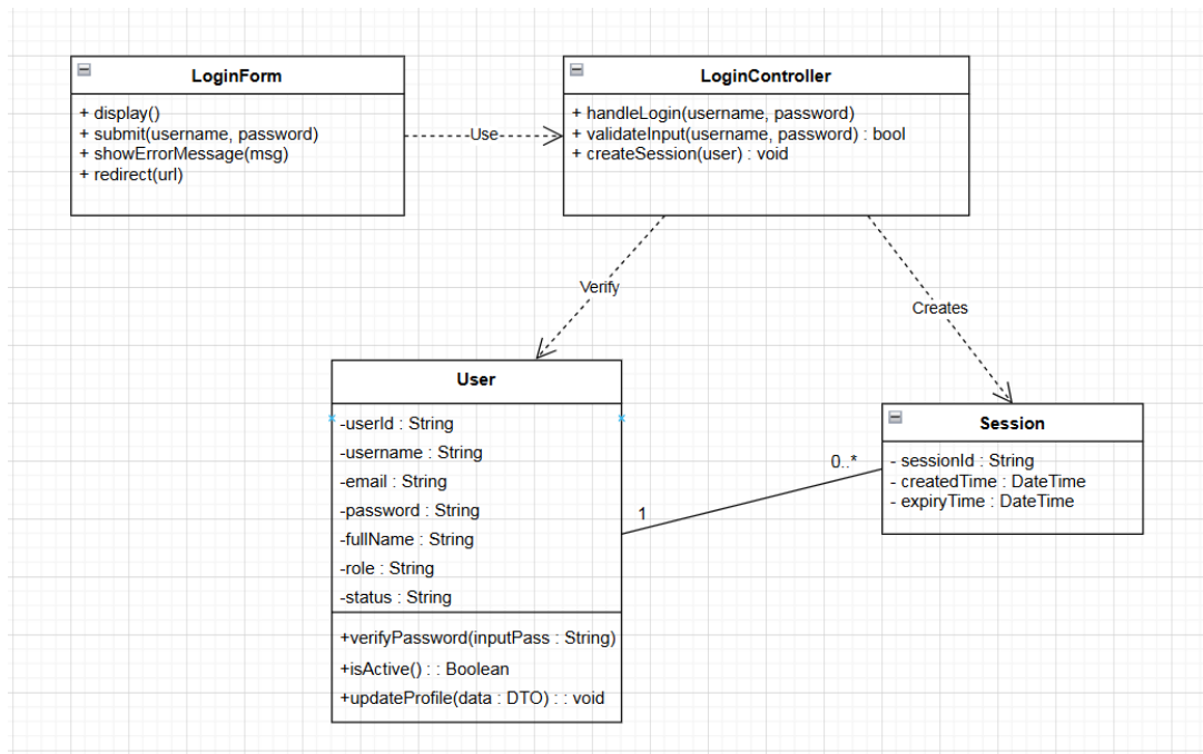
Hình 24: Biểu đồ lớp chi tiết chức năng Đăng nhập
