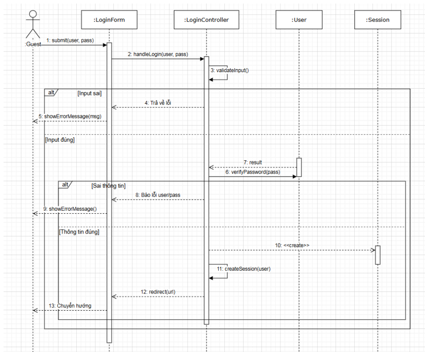
Hình 12: Biểu đồ tuần tự chức năng Đăng nhập
