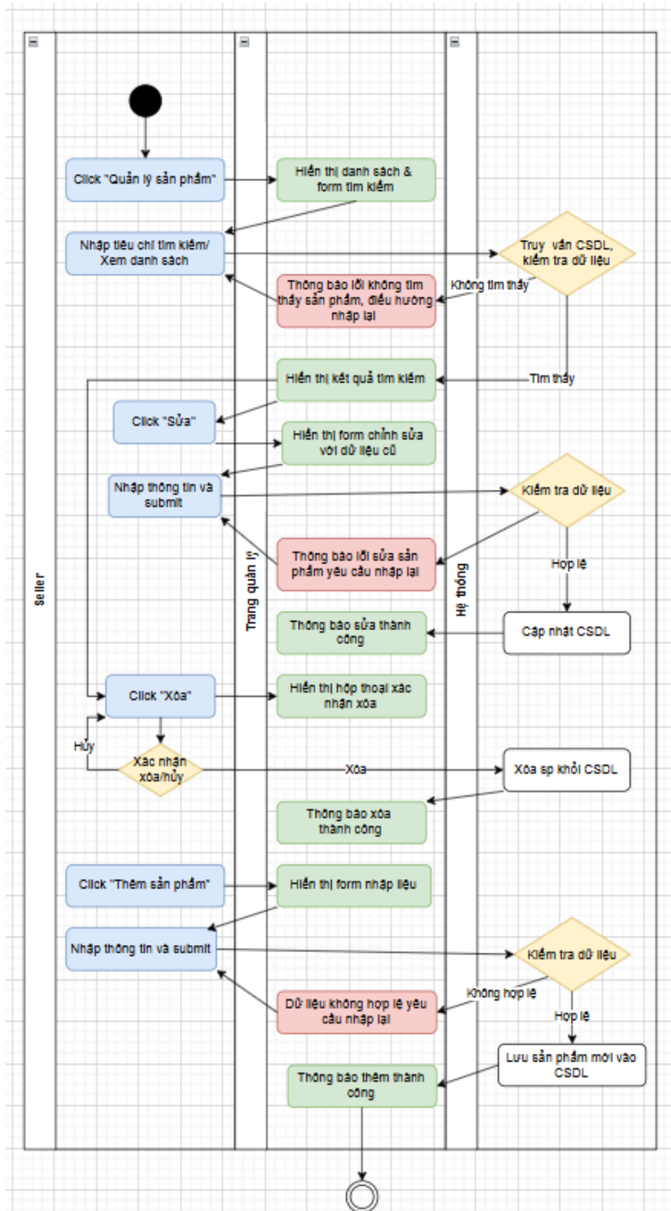
Hình 8: Biểu đồ hoạt động Quản lý sản phẩm của Seller
