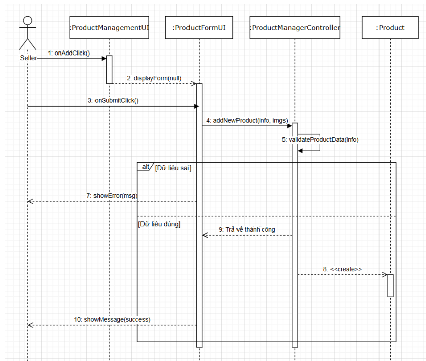
Hình 16: Biểu đồ tuần tự chức năng thêm sản phẩm
