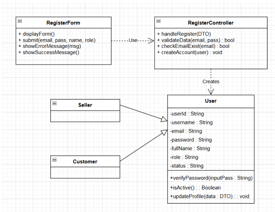
Hình 23: Biểu đồ lớp chi tiết chức năng Đăng ký
