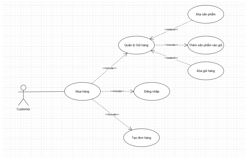
Hình 2: Biểu đồ phân rã Use Case Mua hàng
