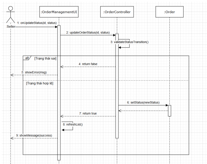
Hình 19: Biểu đồ tuần tự chức năng quản lý đơn hàng
