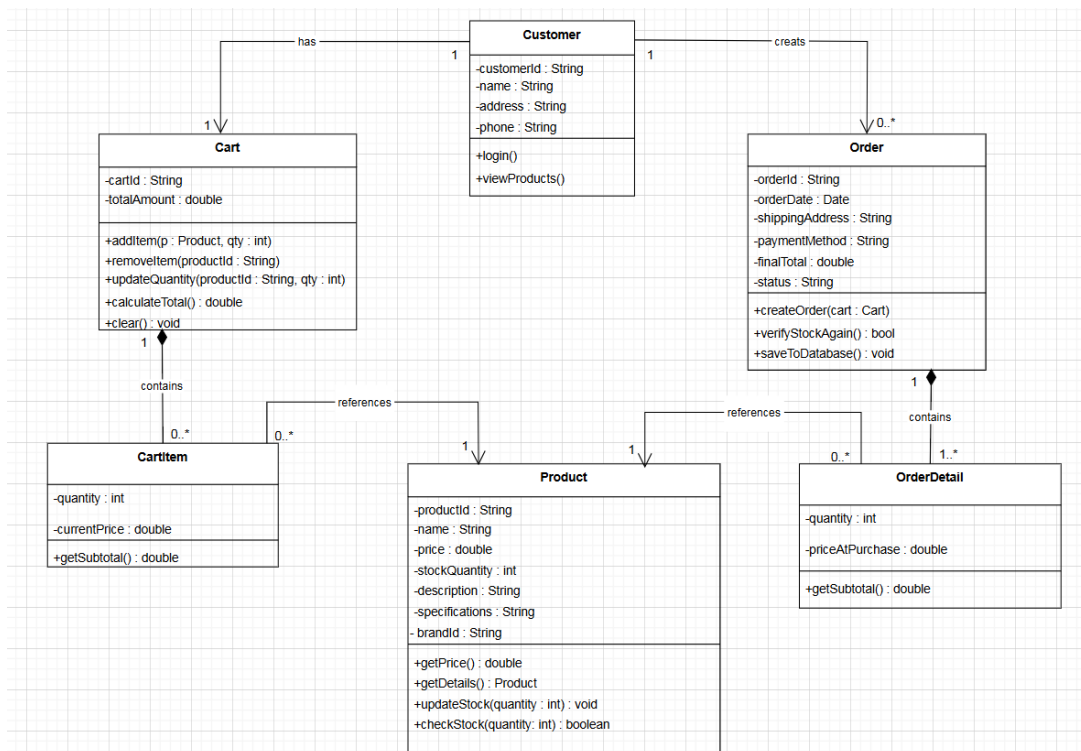
Hình 25: Biểu đồ lớp chi tiết chức năng Mua hàng
