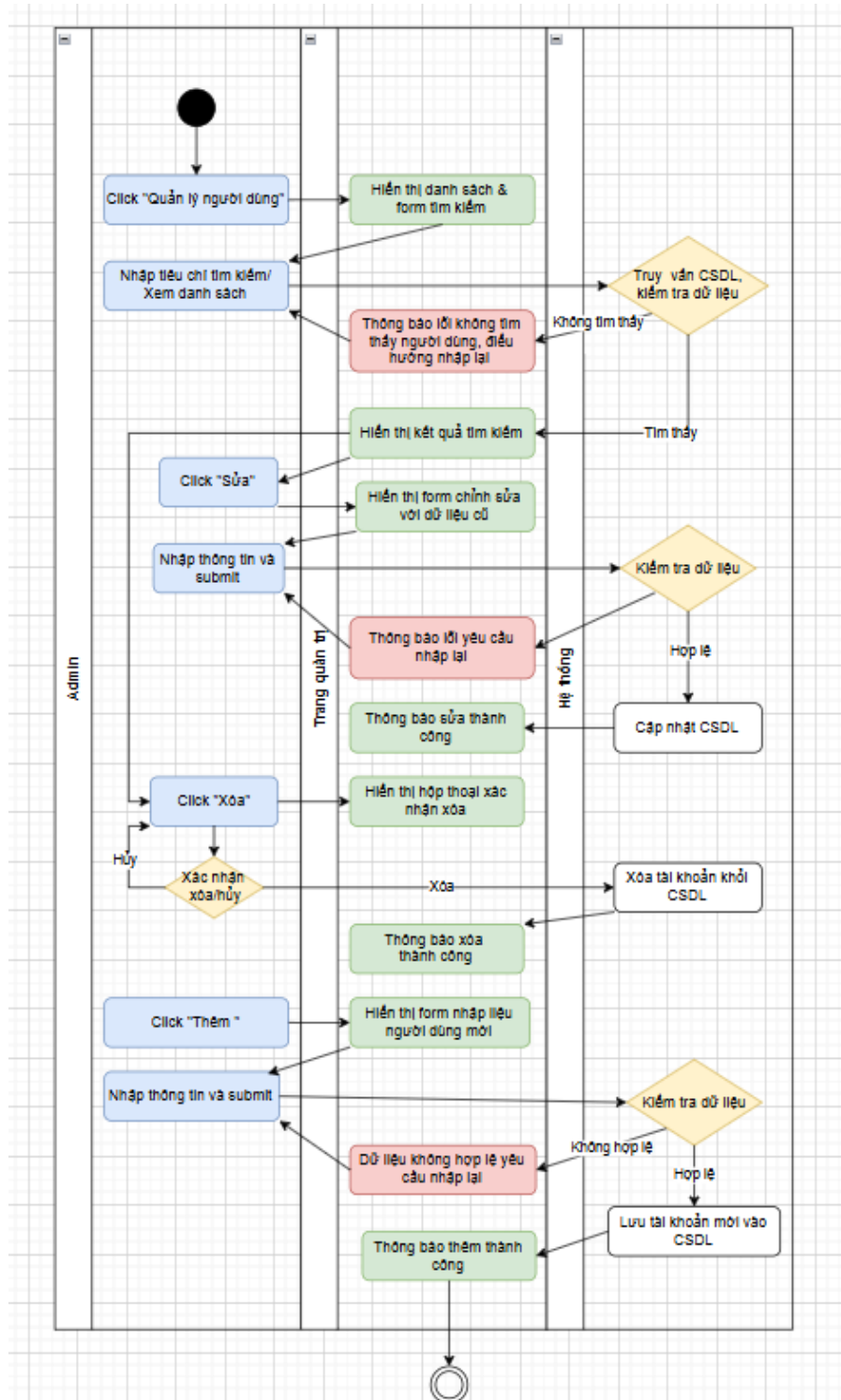
Hình 10: Biểu đồ hoạt động Quản lý người dùng của Admin
