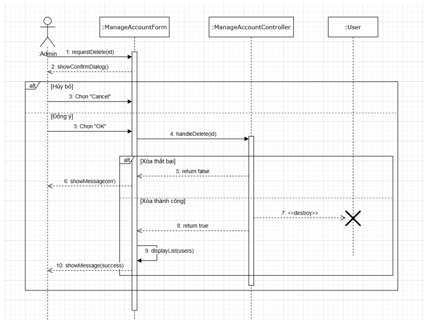
Hình 21: Biểu đồ tuần tự chức năng xóa người dùng
