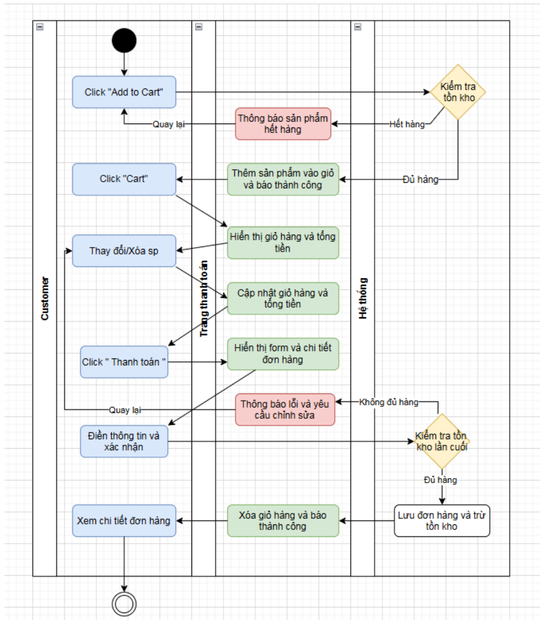
Hình 7: Biểu đồ hoạt động quy trình Mua hàng
