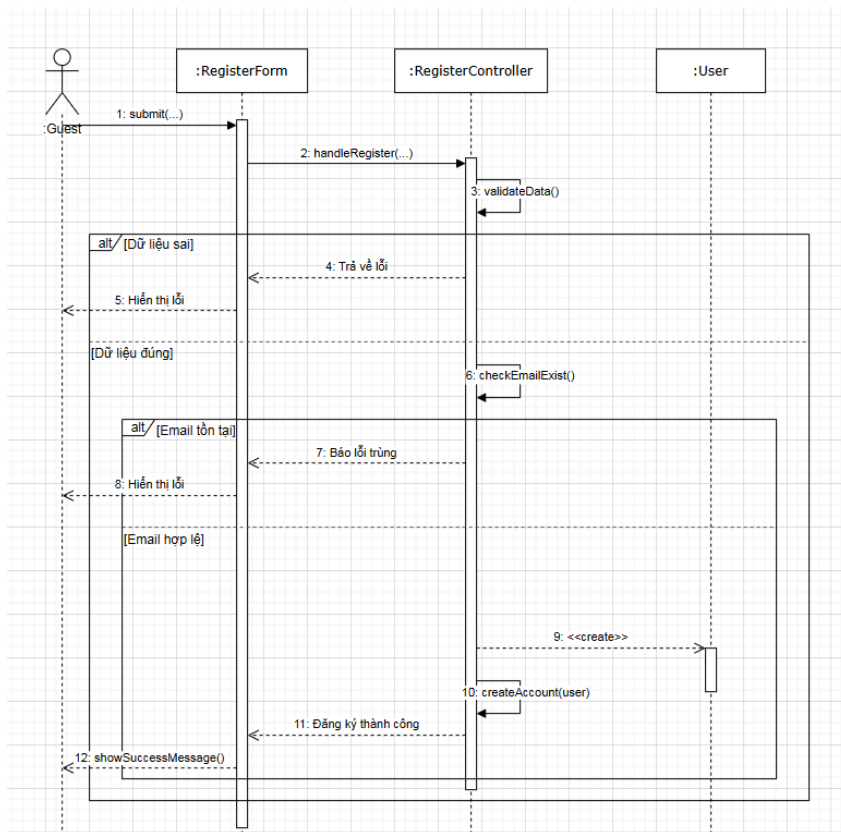
Hình 11: Biểu đồ tuần tự chức năng Đăng ký
