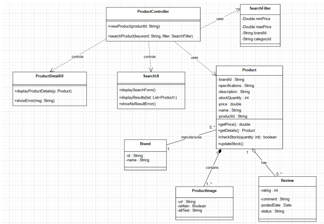
Hình 29: Biểu đồ lớp chi tiết chức năng Tìm kiếm và xem thông tin sản phẩm
