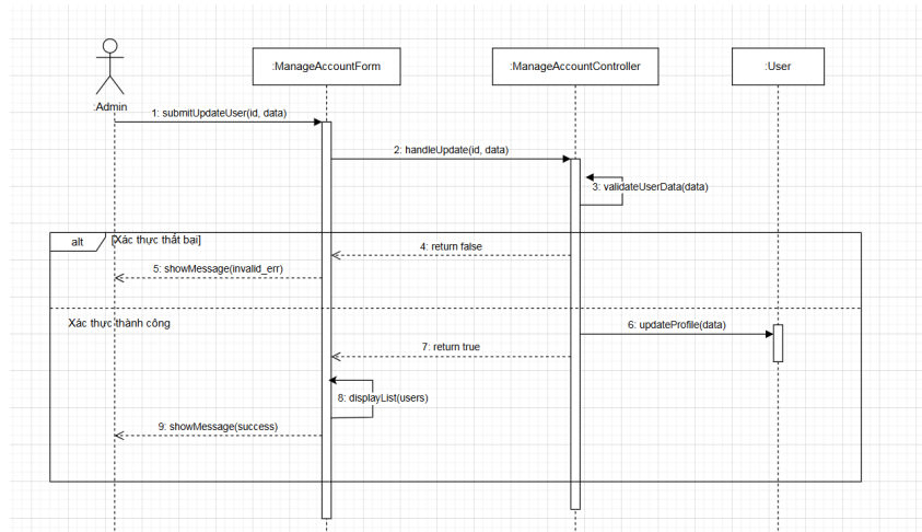
Hình 22: Biểu đồ tuần tự chức năng sửa thông tin người dùng
