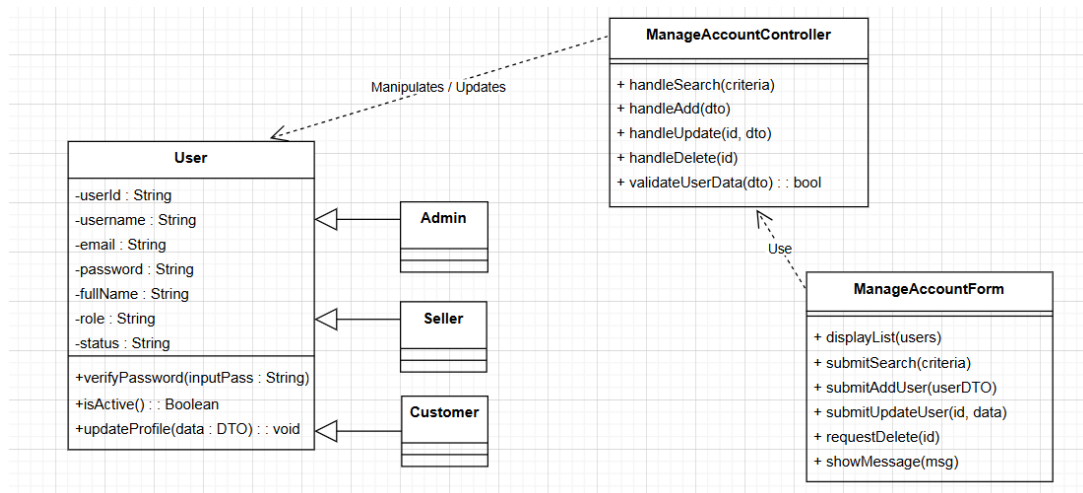
Hình 27: Biểu đồ lớp chi tiết chức năng Quản lý người dùng
