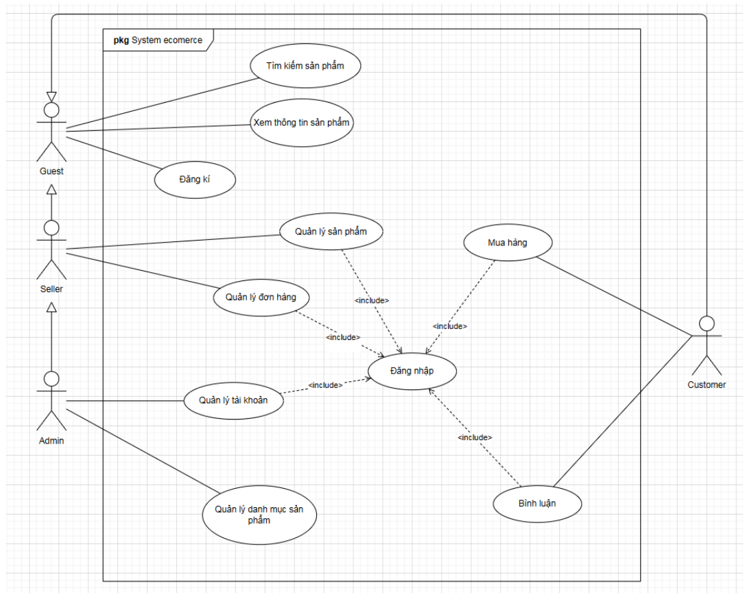
Hình 1: Biểu đồ Use Case tổng quan hệ thống thương mại điện tử
