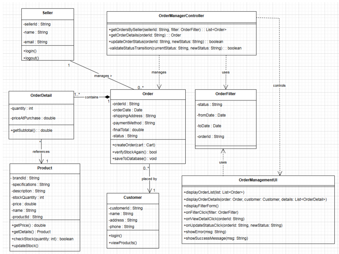
Hình 26: Biểu đồ lớp chi tiết chức năng Quản lý đơn hàng
