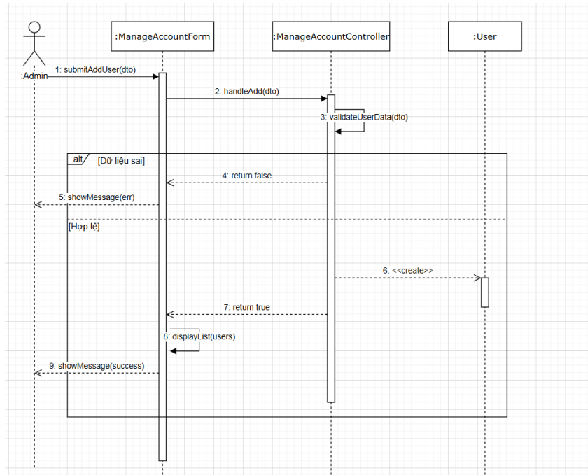
Hình 20: Biểu đồ tuần tự chức năng thêm người dùng
