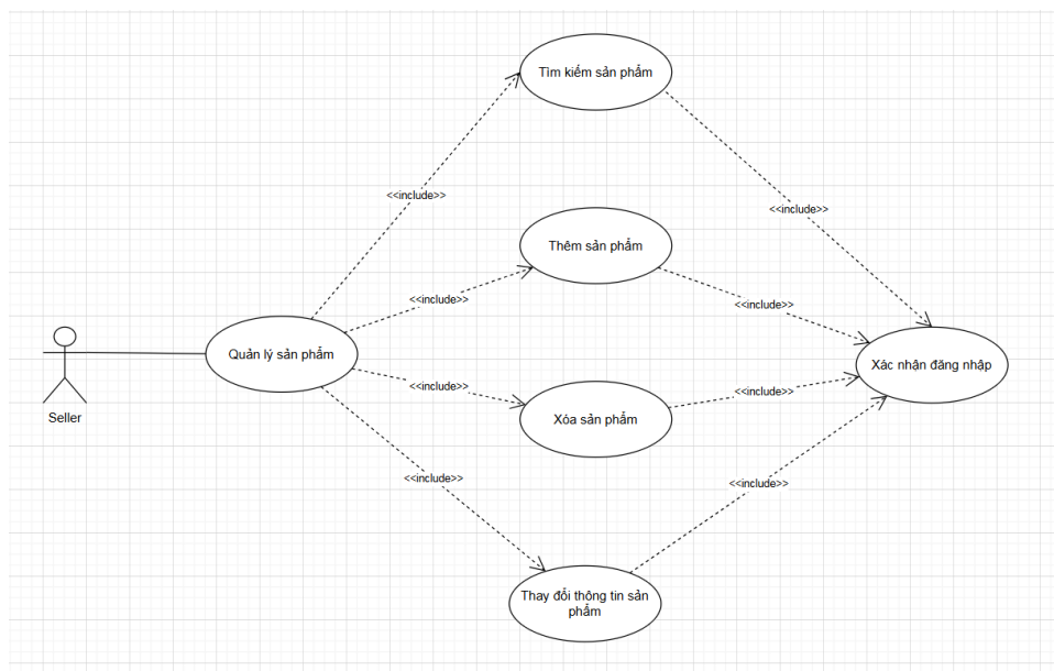
Hình 3: Biểu đồ phân rã ca sử dụng Quản lý sản phẩm
