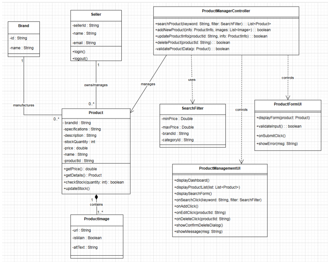
Hình 28: Biểu đồ lớp chi tiết chức năng Quản lý sản phẩm
