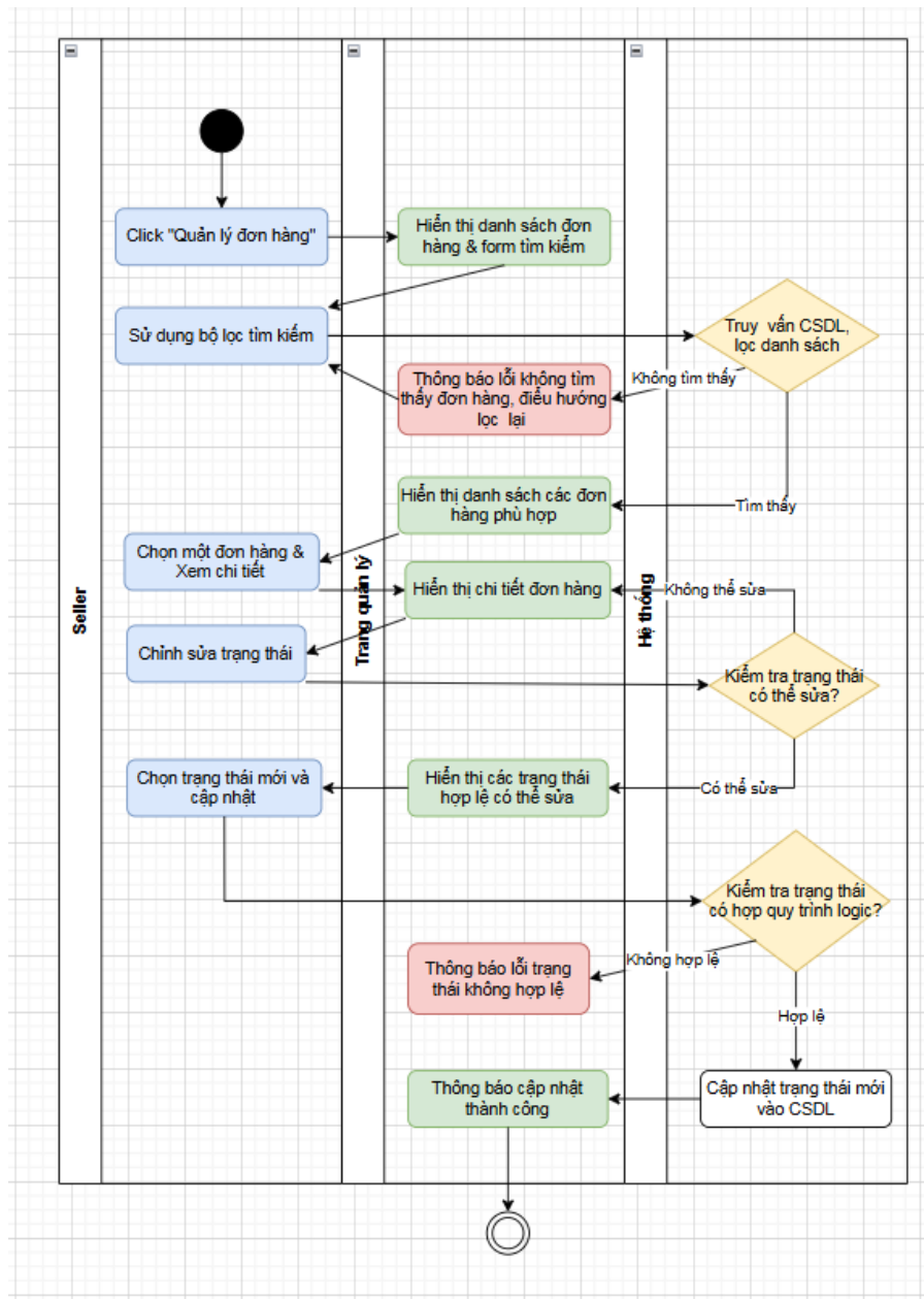
Hình 9: Biểu đồ hoạt động Quản lý đơn hàng của Seller
