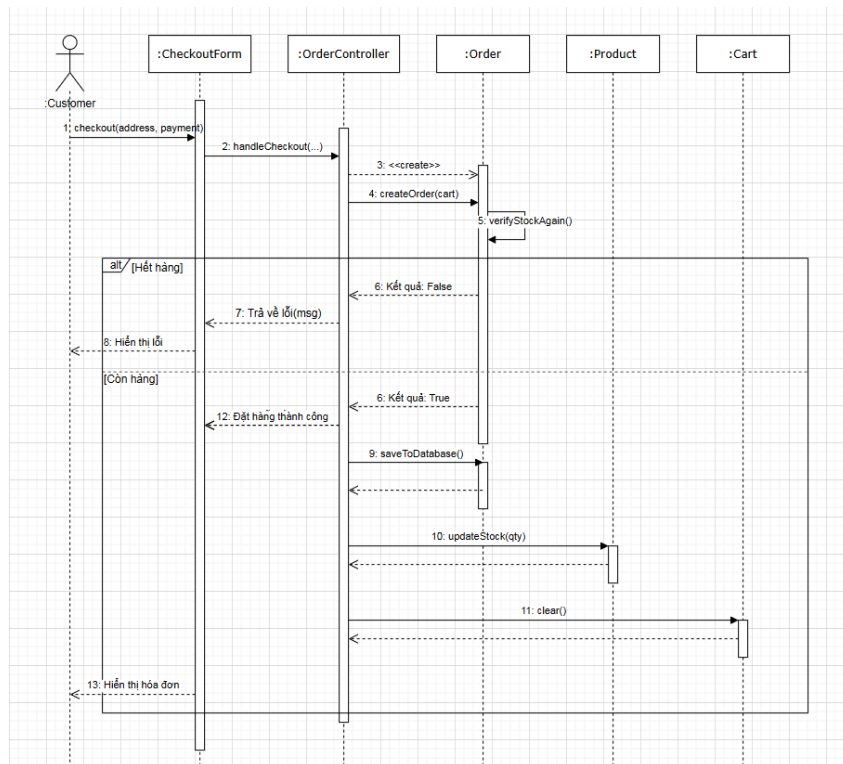
Hình 14: Biểu đồ tuần tự quy trình Mua hàng
