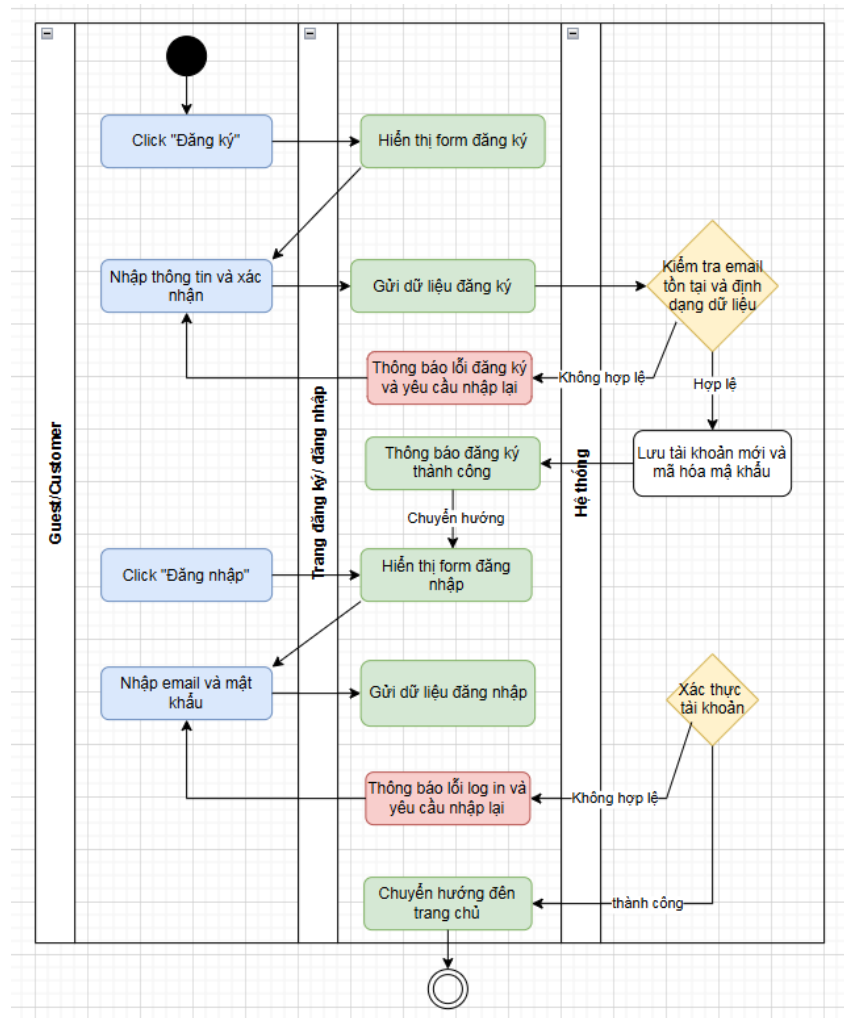
Hình 6: Biểu đồ hoạt động chức năng Đăng ký
