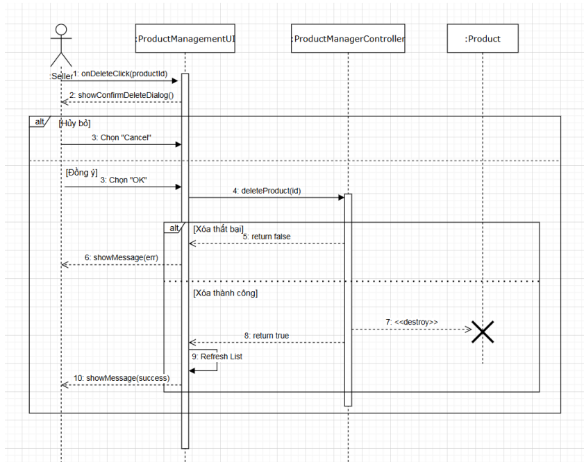
Hình 17: Biểu đồ tuần tự chức năng xóa sản phẩm
