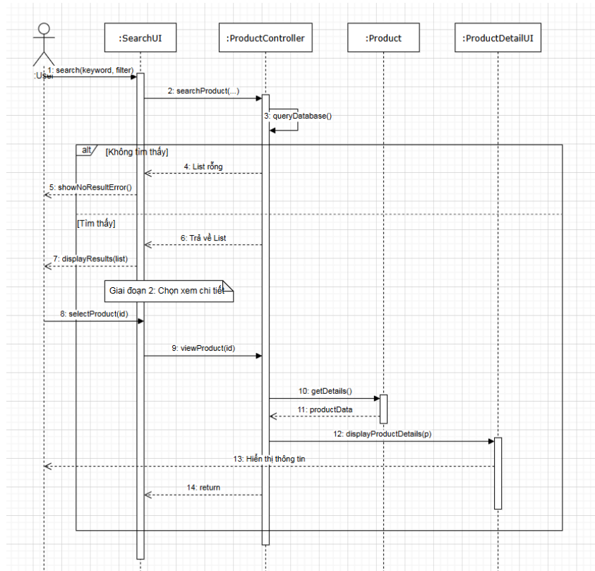
Hình 13: Biểu đồ tuần tự chức năng Tìm kiếm sản phẩm
