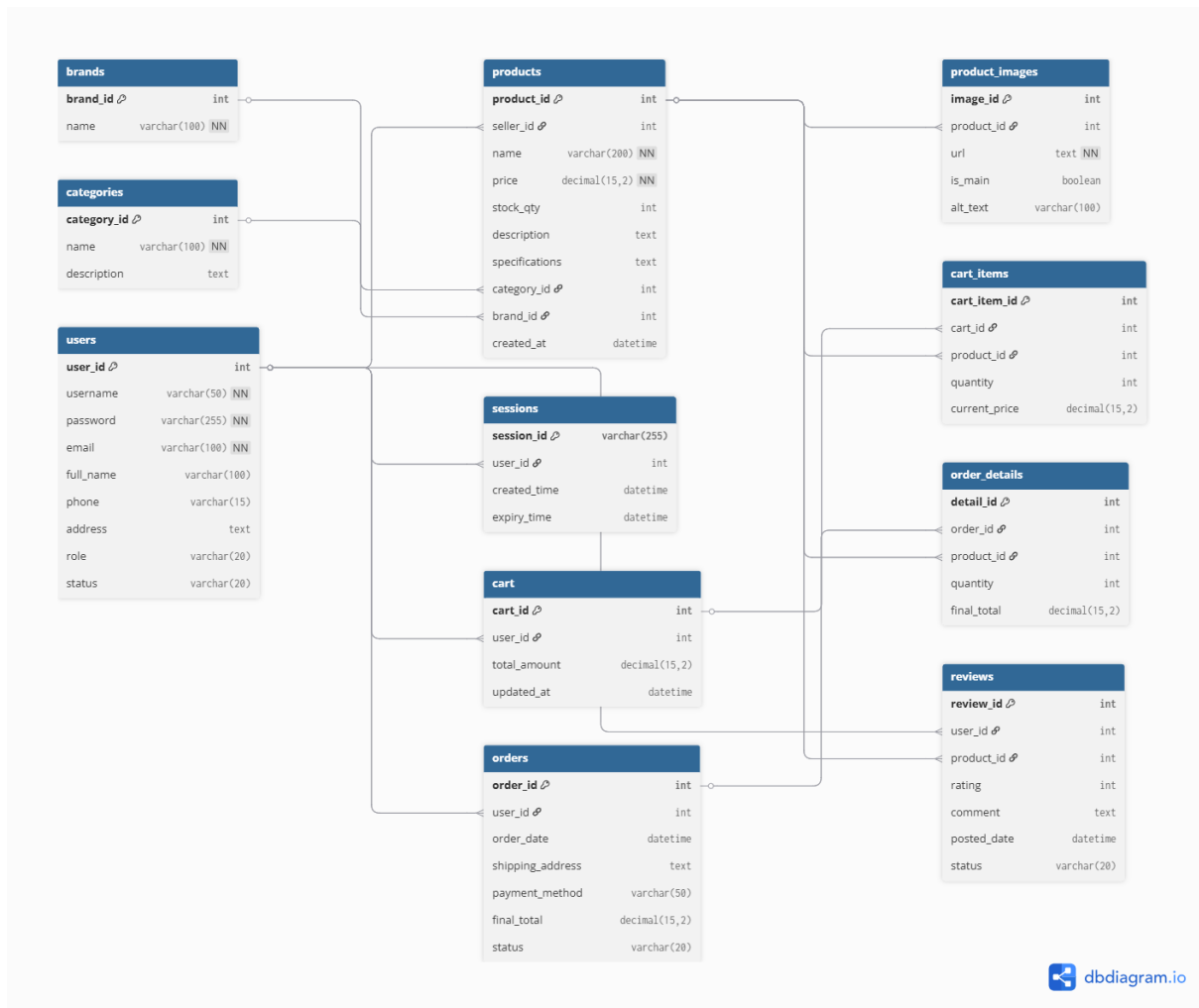
Hình 31: Sơ đồ quan hệ thực thể (ERD)
