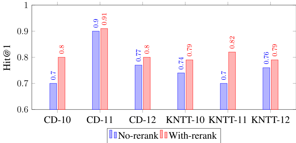
Hình 4.3: So sánh Hit@1 giữa hai cấu hình theo từng nhóm bộ sách và khối lớp
