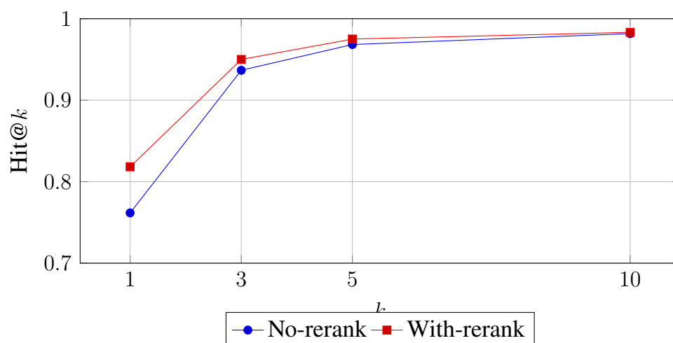
Hình 4.2: Hit@ k theo k của hai cấu hình trên toàn bộ 600 câu hỏi
