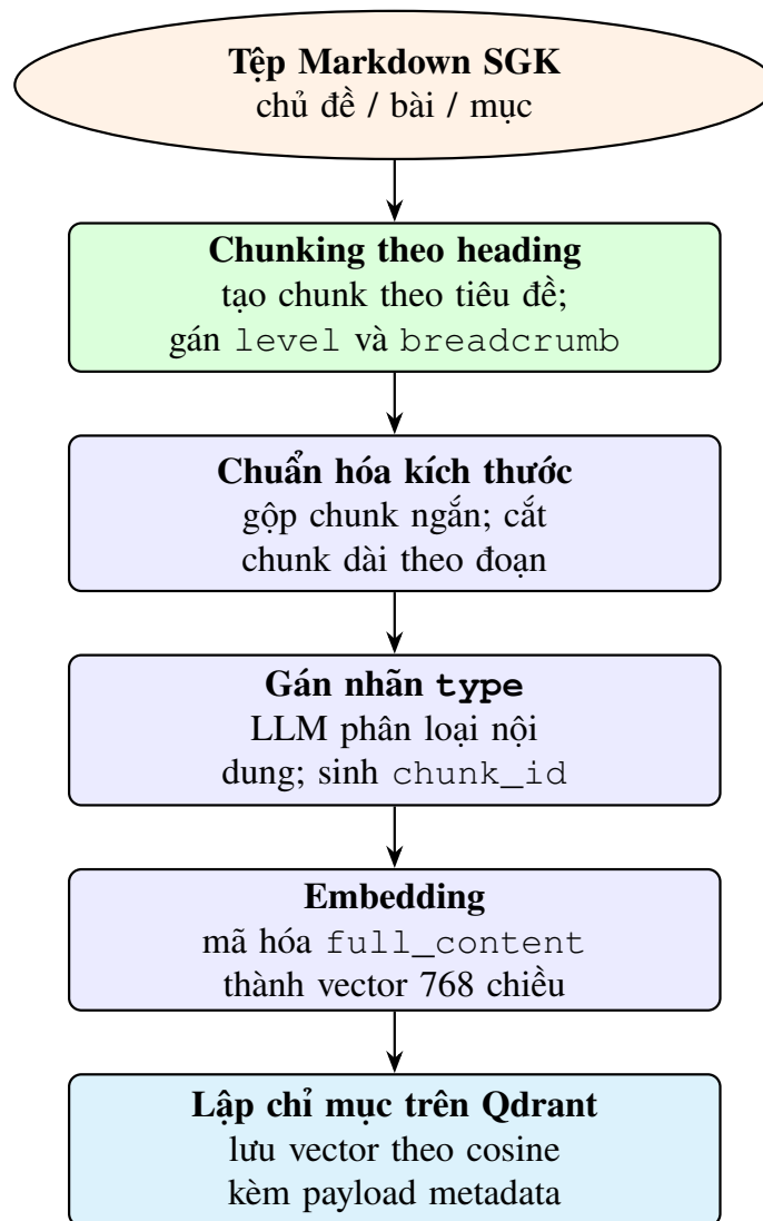
Hình 3.2: Quy trình từ văn bản SGK đến tập phân đoạn được lập chỉ mục, với phân đoạn theo tiêu đề là bước trung tâm
