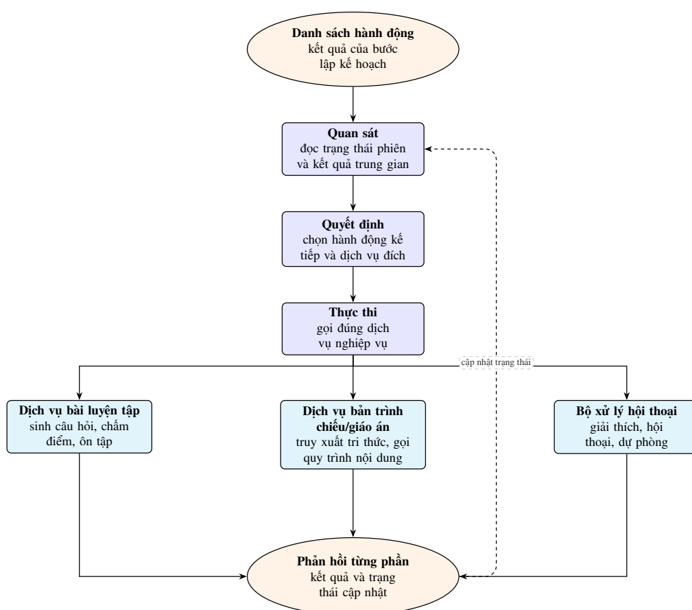
Hình 3.6: Vòng thực thi đa hành động trong tầng điều phối theo chu trình quan sát – quyết định – hành động
