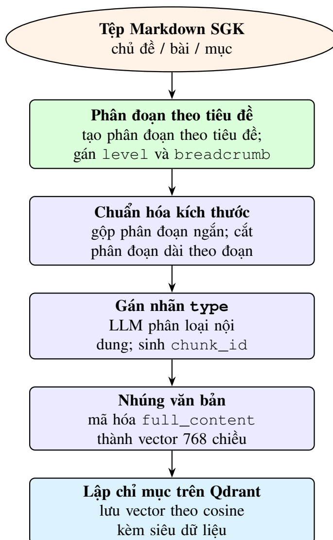
Hình 3.2: Quy trình từ văn bản SGK đến tập phân đoạn được lập chỉ mục, với phân đoạn theo tiêu đề là bước trung tâm
