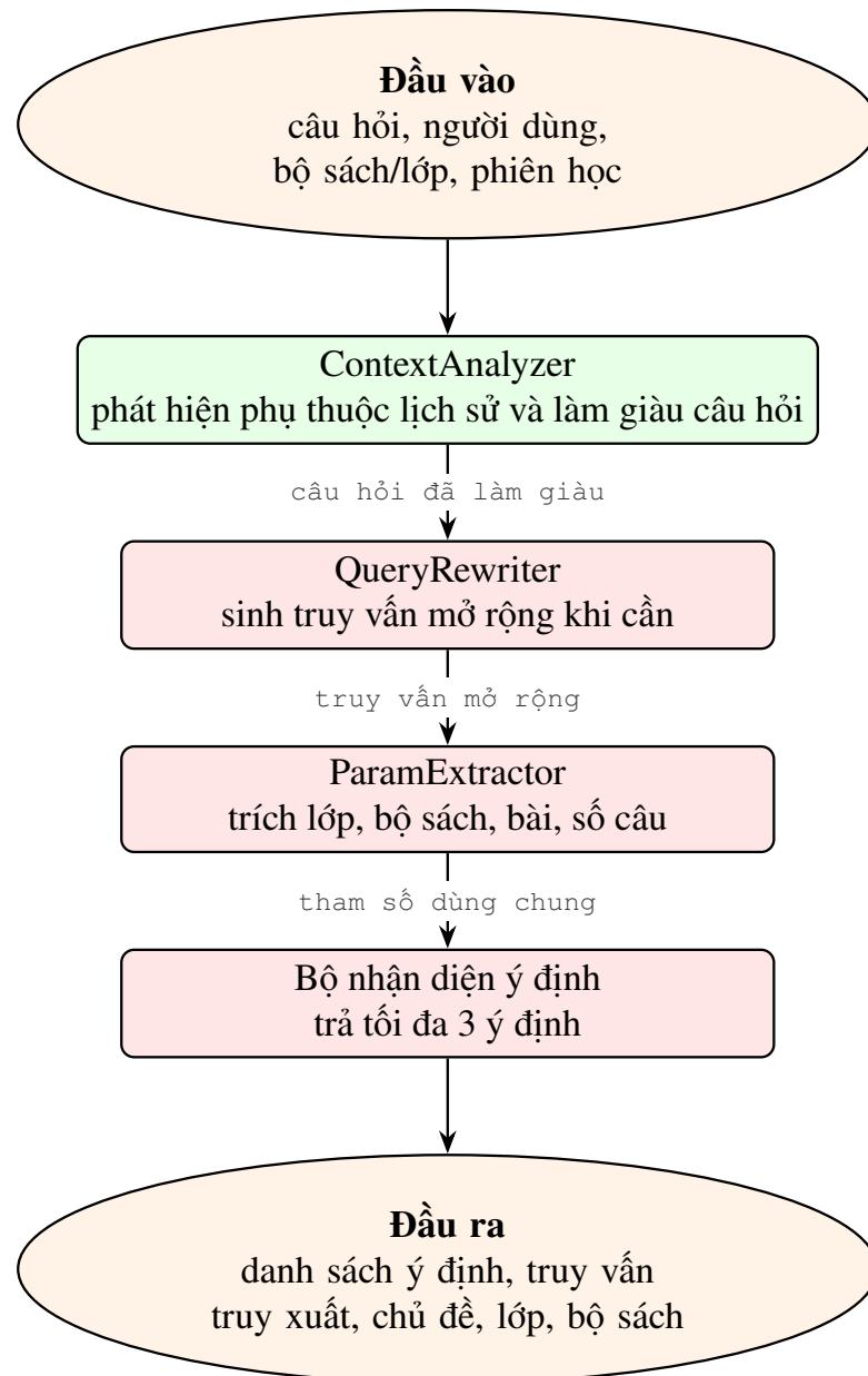
Hình 3.4: Khối phân tích ngữ cảnh và định tuyến ý định trong tầng điều phối
