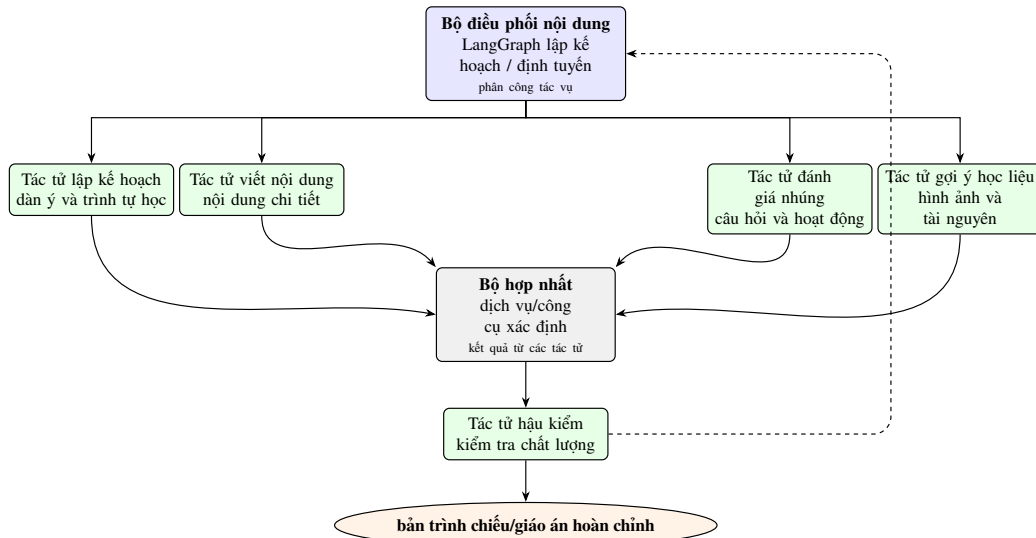
Hình 3.7: Kiến trúc đa tác tử cho bài toán sinh bản trình chiếu và giáo án
