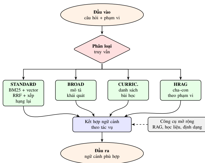
Hình 3.3: Cơ chế truy hồi thích ứng của hệ thống
