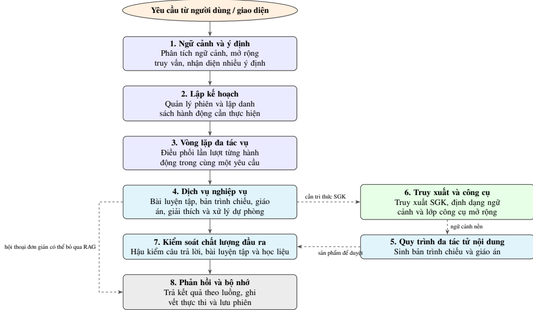
Hình 3.1: Kiến trúc tổng thể của phương pháp đề xuất theo hướng phân tầng, trong đó lõi truy xuất tri thức là nền dùng chung cho các nhánh xử lý
