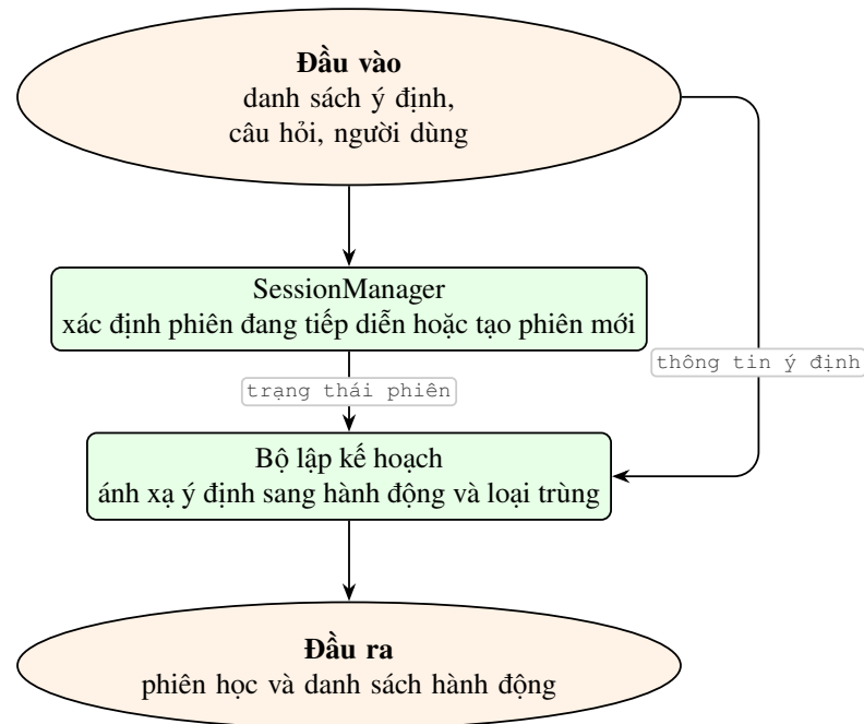
Hình 4.3: Chu trình lập kế hoạch hành động bằng rule-based logic
