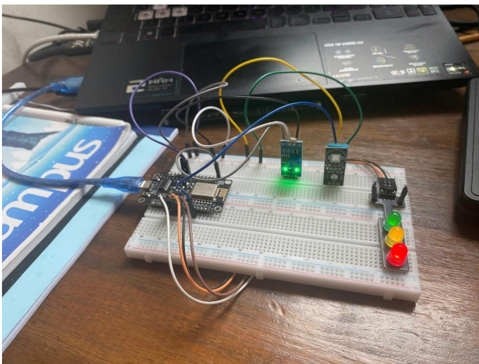
Hình 4.2: Đèn LED ở trạng thái BẬT sau khi nhận lệnh từ Web App
