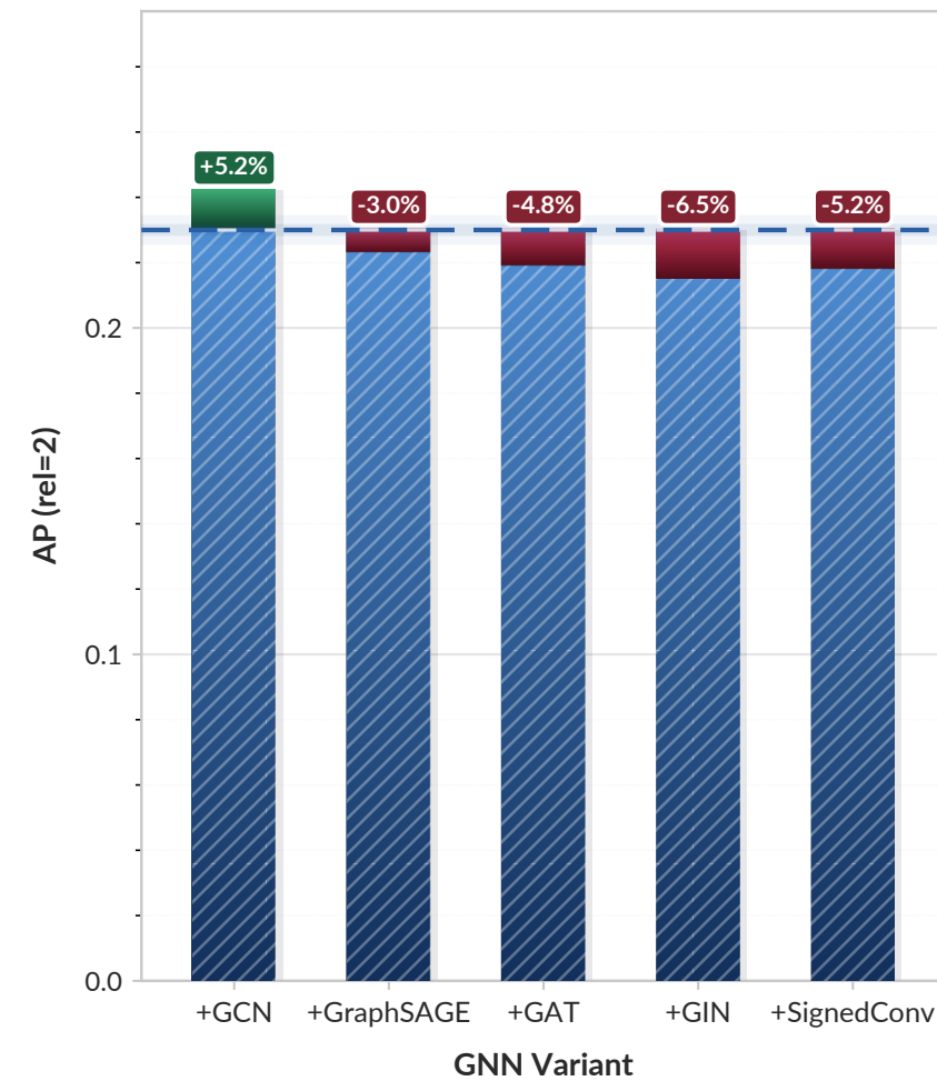
DL-Hard
