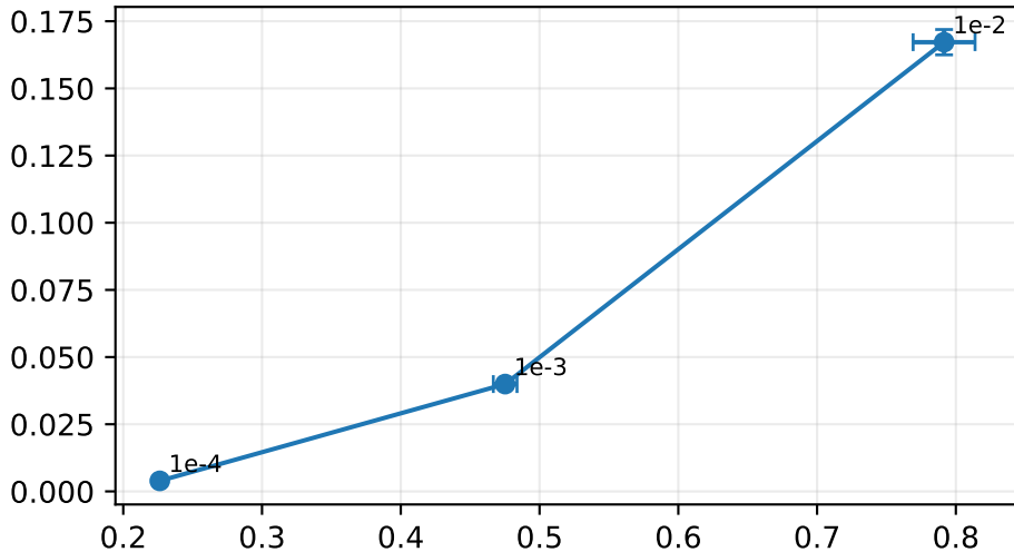
Mean posterior \sigma
