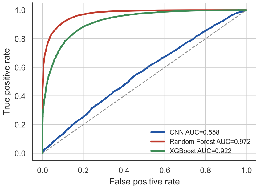
Random-split ROC
