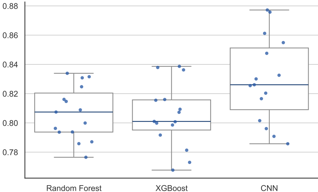
Held-out-run F1
