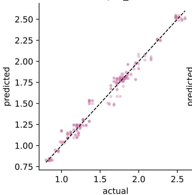
Predicted vs actual on ebw (full context)
