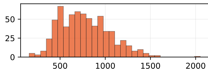
emad
