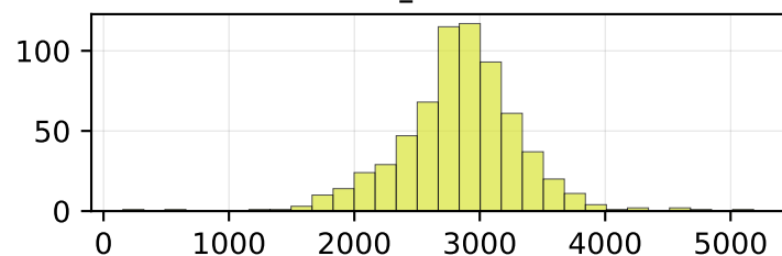
emad
