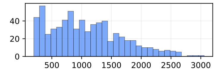
red_edge_3
