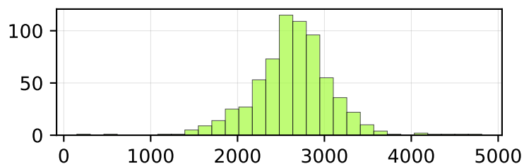
swir_2
