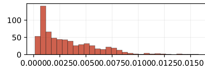
smad
