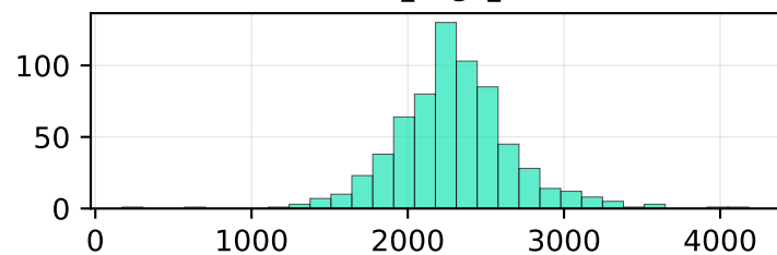
nir_narrow
