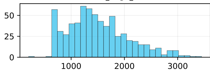
nir
