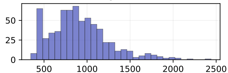
red_edge_2
