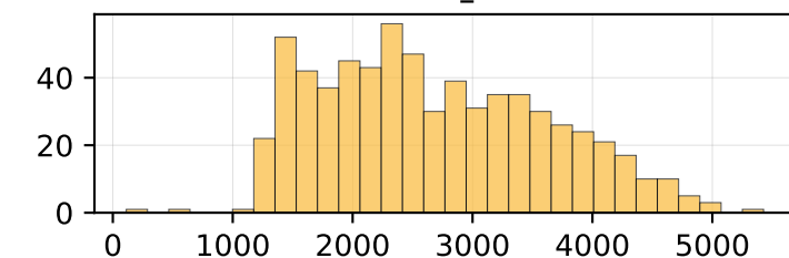
smad
