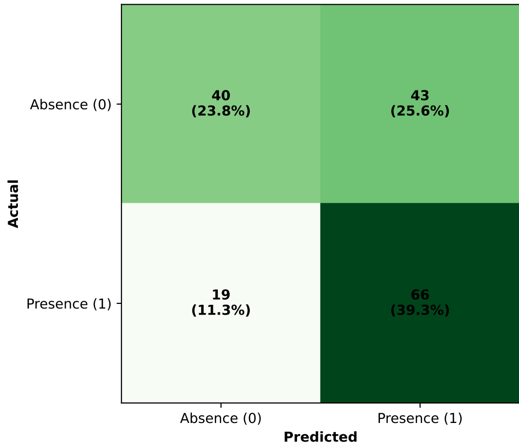
H) Confusion Matrix - TCI
