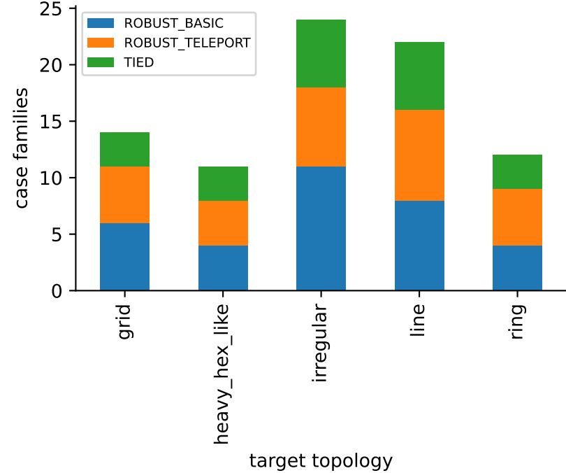
Winner robustness
