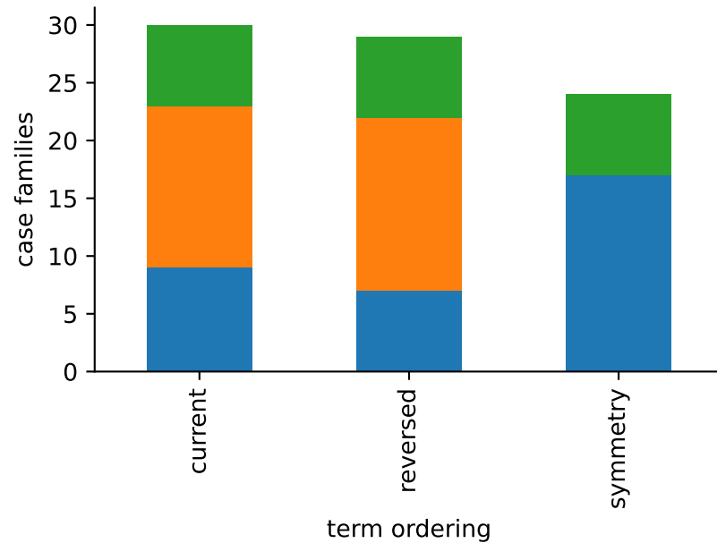
Winner robustness
