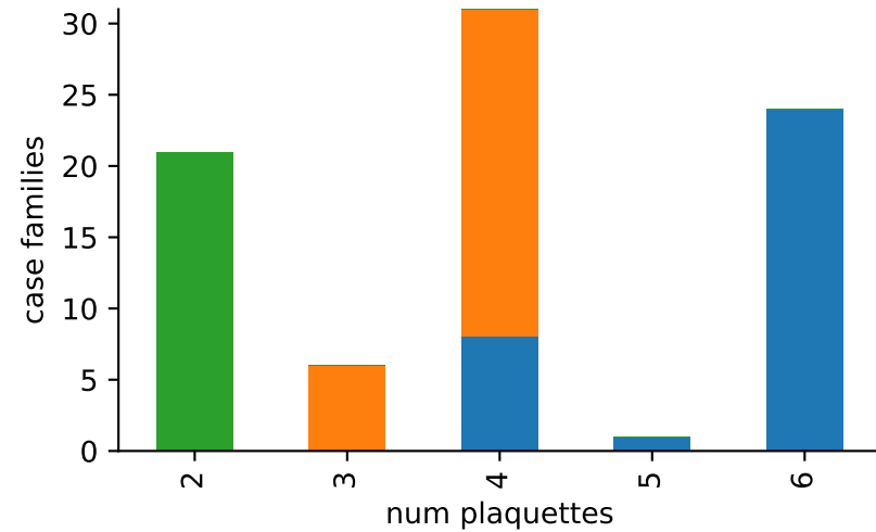
Winner robustness
