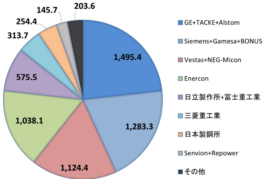
2025年12月末メーカー別累計設備容量 (合計6,434.2MW)
