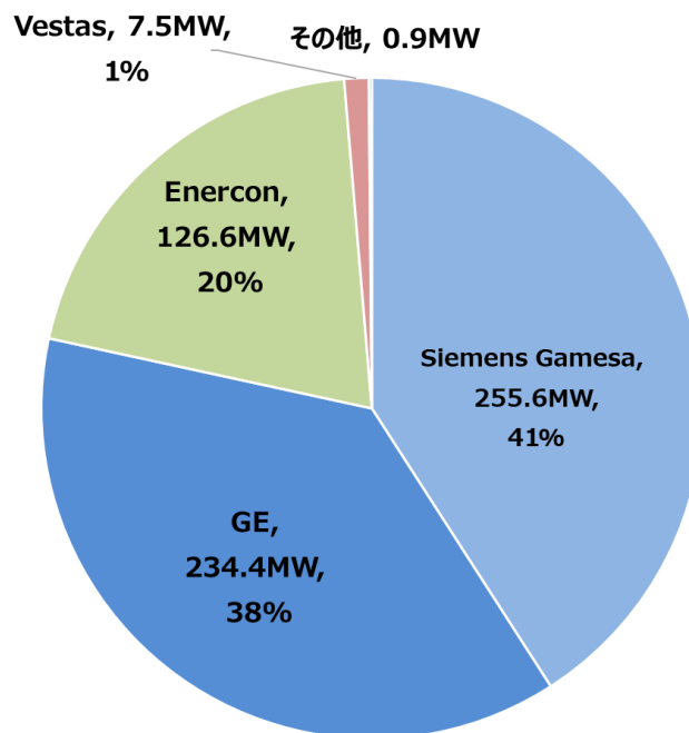
2025年1～12月 新規導入の風車シェア (Grossで計625.0MW)
