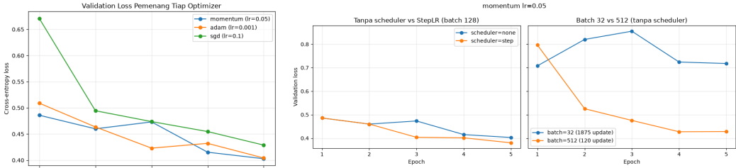
Gambar 2. Validation loss per epoch pada momentum \eta = 0,05 . Kiri: tanpa scheduler vs StepLR (batch 128). Kanan: batch 32 vs 512 tanpa scheduler, dengan jumlah update di legenda.
