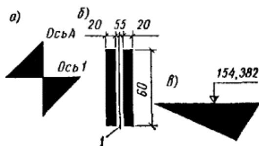
Рис. 15. Откраска осей (а, б) и отметок (в) на конструкциях зданий и сооружений
