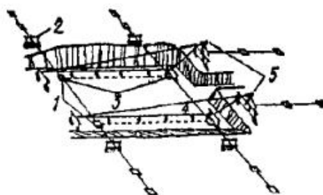
Рис. 8. Перенос разбивочных осей на дно котлована
