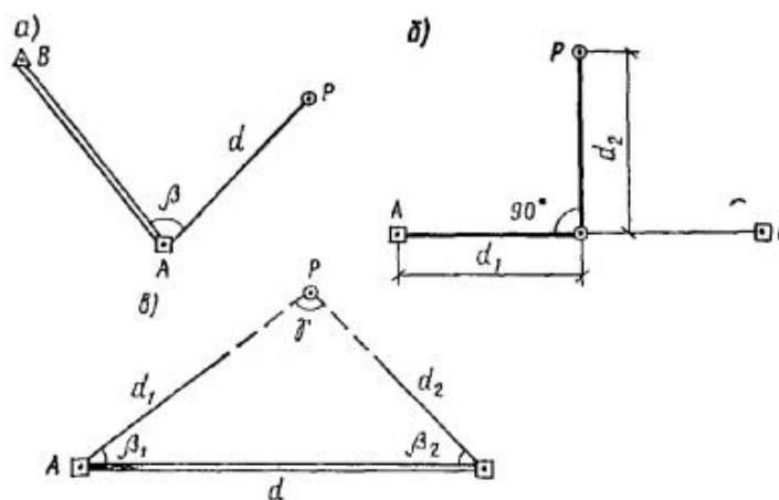
Рис. 3. Способы разбивки точек сети
