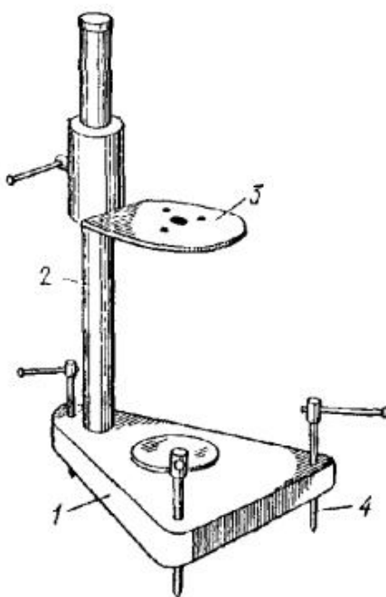
Рис. 6. Консольный штатив для установки геодезических приборов
