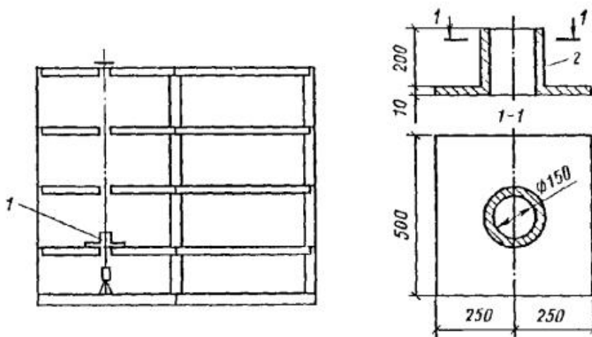
Рис. 16. Ловушка, схема ее установки
