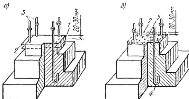
Рис. 11. Подготовка фундамента для монтажа стальных колонн
