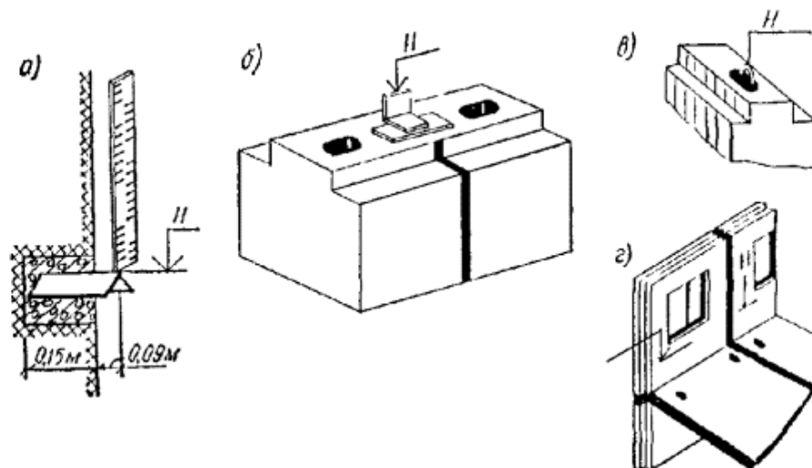
Рис. 17. Знаки закрепления высотной разбивочной сети
