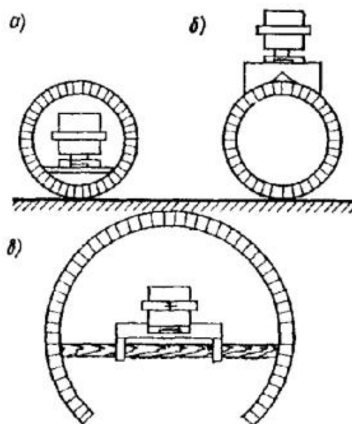
Рис. 5. Установка навесных контрольных марок на секции трубопровода
