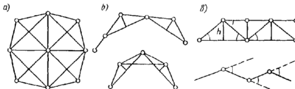
Рис. 13. Схемы внутренних разбивочных сетей зданий и сооружений
