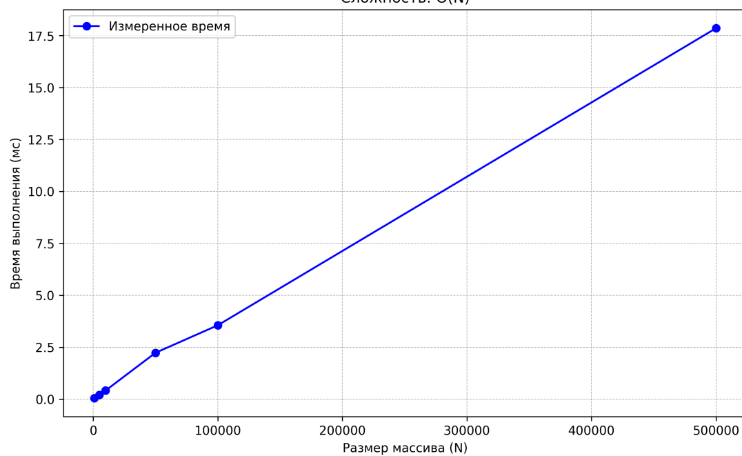
Зависимость времени выполнения от размера массива Сложность: O(N)
