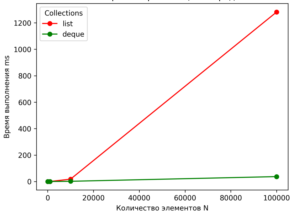
Тест времени реализации очереди
