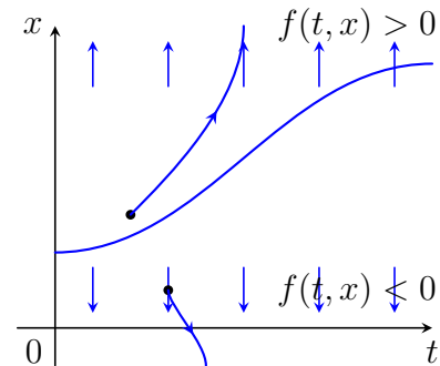
Рисунок 2 — Пример неустойчивого решения вырожденного уравнения f(t, x) = 0
