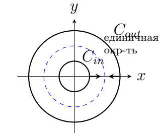
Направление векторного поля на окружностях C_{in}, C_{out}
